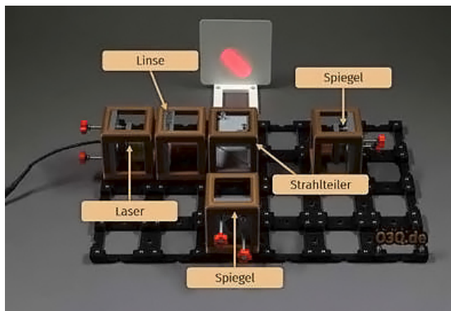
Figur 2. Eksperimentel realisering af Mach-Zehnder-interferometer. Dette byggesæt, der er opbygget af 3d-printede elementer, udgør en fleksibel basis for at gennemføre mange af de eksperimenter, som er relevante for behandling af fotoners egenskaber. Udstyret er udviklet ved Universitetet i Münster / Nils Haverkamp.
