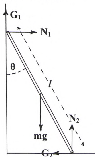
Figur 1. Bræt skråtstillet imod væg.
