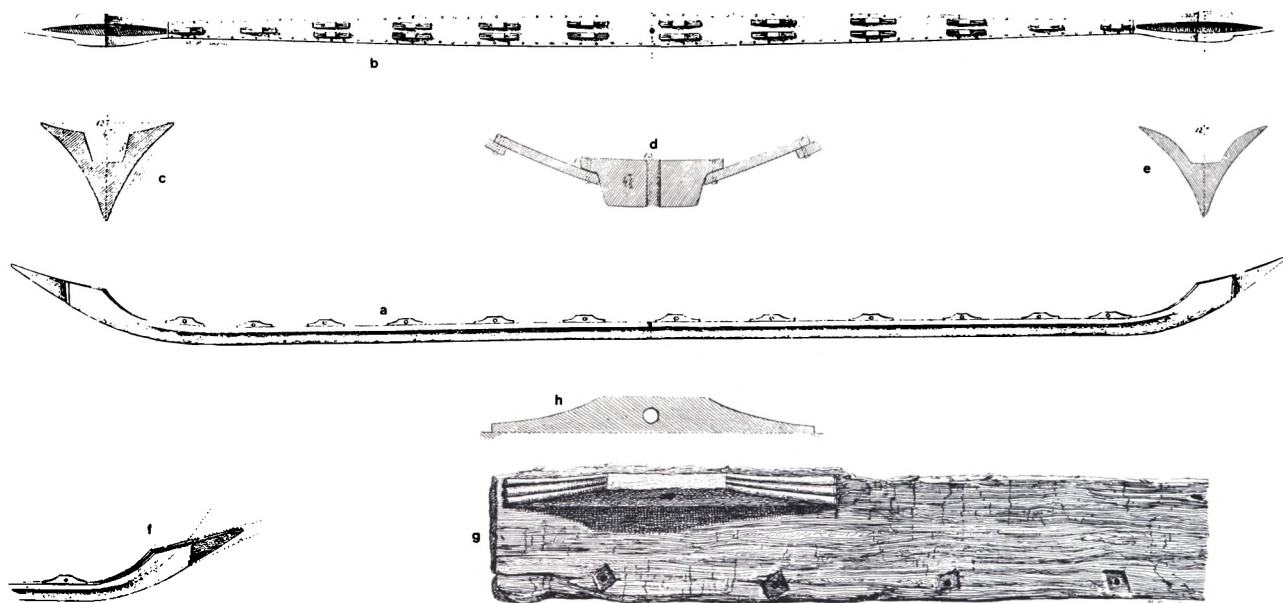
Fig. 3: Fragmenter af fyrretræs båden uden målestoksangivelse. Den udgravedes under Frederik VII's besøg i Nydam den 27. oktober 1863. Efter Engelhardt 1865. Båden er ifølge overleveringen blevet efterladt på en mark nær mosen tildekket med mosejord, medens man tog sig af egetræs bådens opstilling. På grund af krigen i 1864 og deraf følgende begivenheder fik Engelhardt ikke mulighed for at tage sig af fyrretræs båden, der således var overladt til ødelæggelse.
