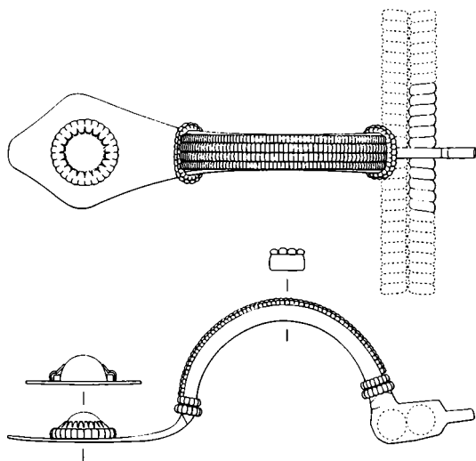
Fig. 3. Rekonstruktionstegning af Foulum-fiblen. Tegning: Orla Svendsen. Mål: 1:1.
