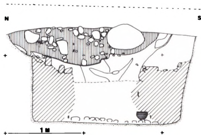
Fig. 3: Tverprofil af grav I og II. Nederste del af grav II konstrueret på grundlag af planopmålinger. Lodret skravering = bopladspræget fyldjord i grav I. Skrå skravering = stenramme i grav II. Kraftige sorte streger = kistespor. Tegning: J.AA.J.
