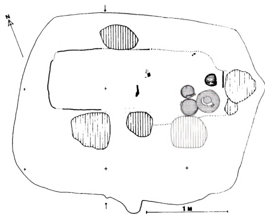
Fig. 1: Plan af grav I. 1) grænse for fyldskifte grav I og II. 2) store støttesten for plankekiste 3) gravbund 4) gruppe af lerkar 5) jernkniv 6-7) ubestemmelige jernfragmenter (Tegning J.Aa.J.).
