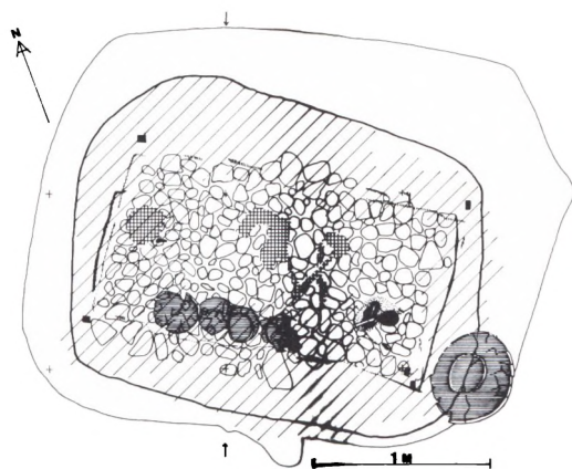
Fig. 5: Plan af grav II. 1) grænse for fyldskifte grav I og II. 2) grænse for nedgravning ved bunden af II. 3) skråskravering = stenrammens største udbredelse. 4) kistespor i to let afvigende niveauer ved gravbunden. 5) pæleaftryk ved kistehjørner. 6) bundbrolægning. 7) 4 lerkar på gravbunden. 8) lurfad og skål oven på nedgravningens sydøst-hjørne. 9) fibula. 10) sammenrustede jerngenstande: saks, kam, kniv m. hornskaft, halvrund kniv. 11) rest af dyreskind, 12) skeletspor. Tegning: J.AA.J.
