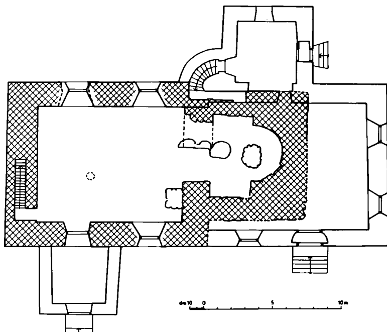
Fig 8. Dörby kyrka. Medeltidskyrkans kor påträffat 1953. Uppmätning Nils Carlgren. Tolkning Karin Andersson. Renritning Kerttu Palmgren 1982.
