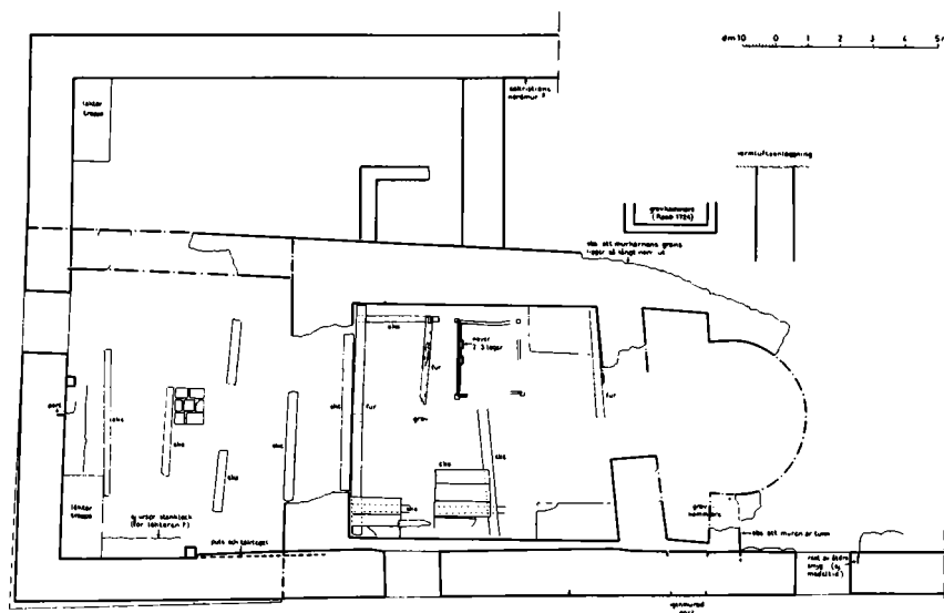
Fig 6. Torsås kyrka. Uppmätning av Iwar Andersson 1956.
