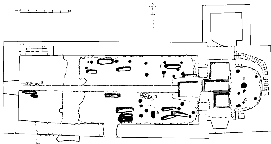
Fig 7. Arby kyrka. Undersökningen 1971-72. Uppmätning Karin Andersson. Renritning Kerttu Palmgren 1977.
