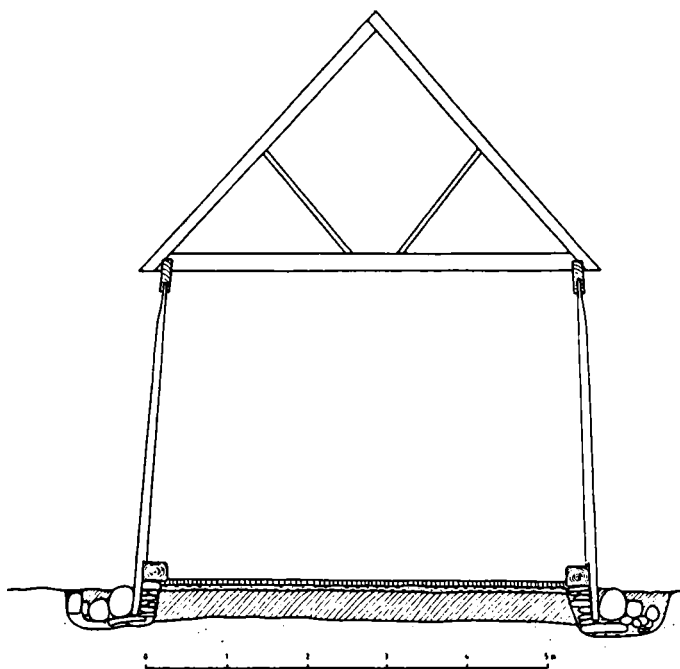
Fig 4. Silte stavkyrka, försök till rekonstruktion av väggar och takstol samt av syll och grundstenar. Efter G Trotzig.
