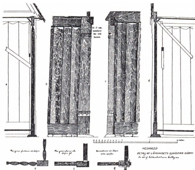
Fig 8. Hedareds stavkyrka, detalj av långhusets sydöstra hörn. Efter E Ekhoft.
