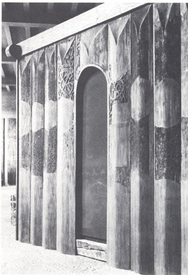
Fig 1. Hemse stavkyrka, västfasaden rekonstruerad i Statens historiska museum, Stockholm. Foto S Hallgren 1963.
