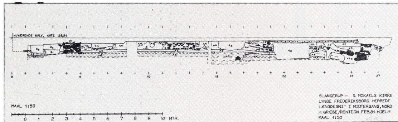
Fig. 5. Sct. Mikæls kirke i Slangerup. Udgravningssnit, H. Græbe 1978.
