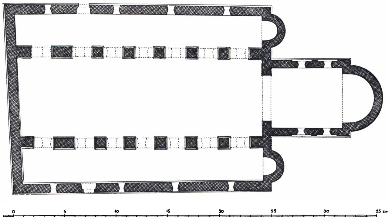
Fig. 1. Roskilde Vor Frue kirke. Rekonstruktionsplan, undersøgt og tegnet af C.G. Schultz 1933-34.
