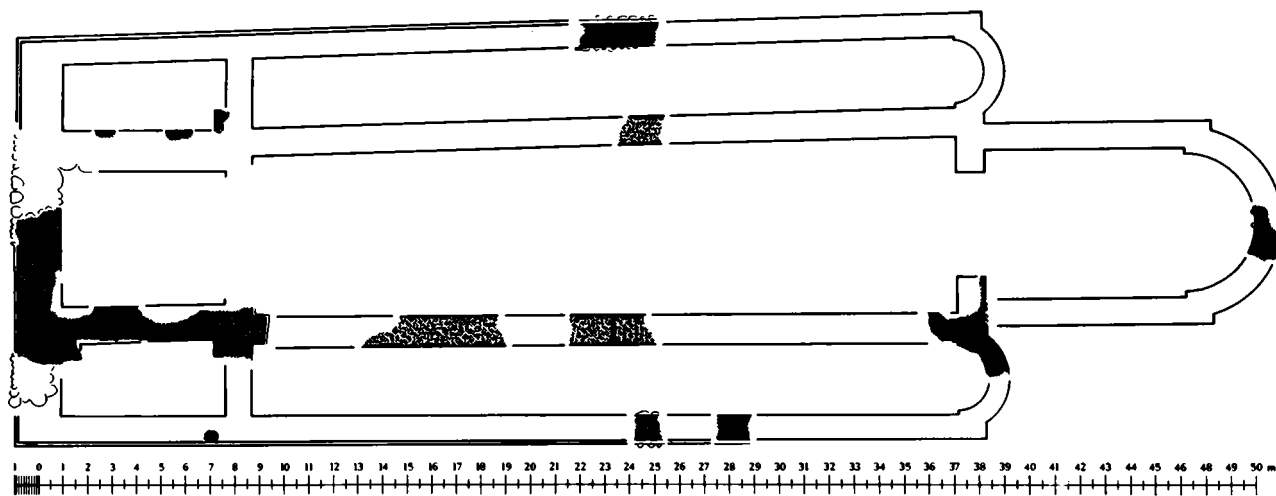
Fig. 3. Erik Ejegods kirke i Slangstrup. Rekonstruktionsplan. Undersøgelser 1936, 1945 og 1973. Tegnet af Elna Møller 1973. Vedrørende østpartiet står spørgsmålet om korets nøjagtige længde åbent, såvel som der er uklarhed om apsidens bredde i forhold til koret. Foruden de krydsskraverede partier er den nøjagtige placering og tykkelse af søndre kormur kendt på det sted, hvor den støde op til triumfmuren.
