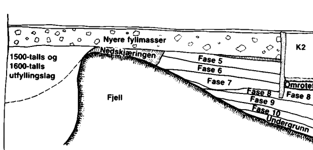
Fig. 2b. Skjematisk fremstilling av feltets stratigrafi i snitt.
