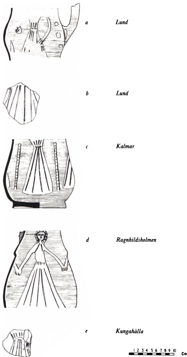
Fig. 3. Skår af dansepigekander fundet i Sydsvrige. Efter Barton 1968a.
