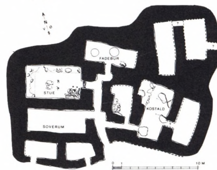
Fig. 1. De tre typer eksemplificeret ved grundplanerne fra 1: Sandnæs. V51, 2: Ø2 og 3: Nipaitsoq V54. 1 og 2 efter Roussell 1941.
