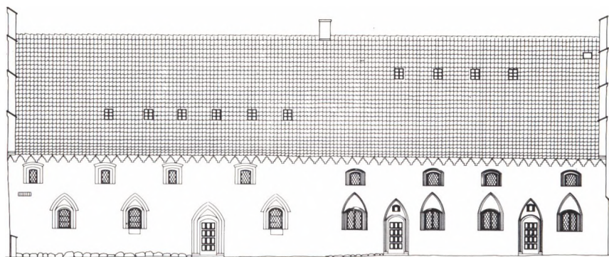
Fig. 1. Helligåndshusets sydside (længde 33,5 m).
