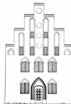
Fig. 4. Helligåndshusets vestgavl (bredde 9,4 m, højde 14,0 m).
