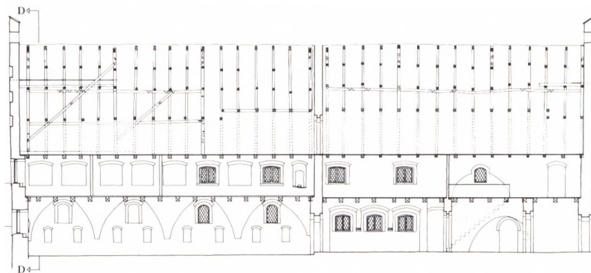
Fig. 3. Længdesnit, set mod nord.
