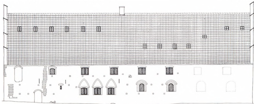
Fig. 2. Helligåndshusets nordside (længde 33,5 m).
