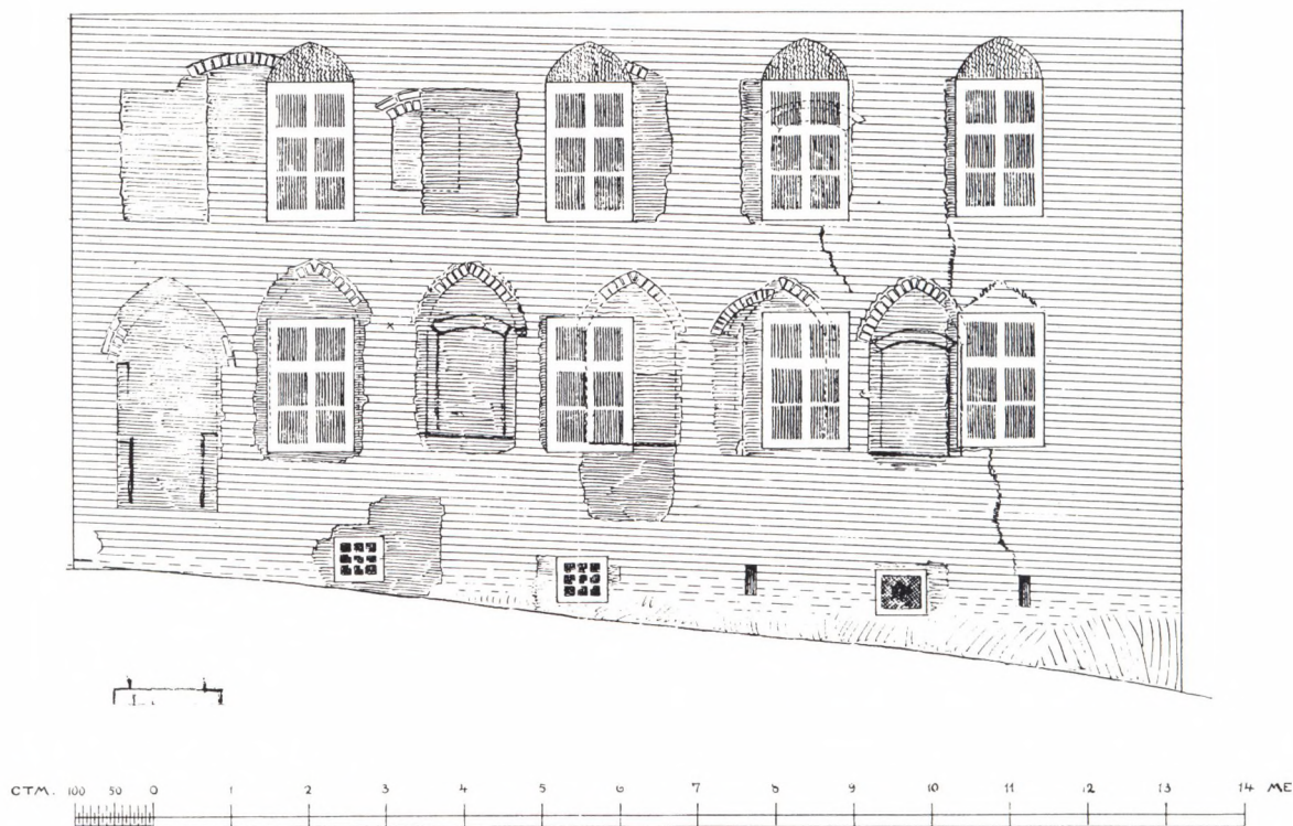
Fig. 4. Opstalt af sydsiden før restaureringen. Bemærk de fladbuede stik fra de senere indsatte, lidt større vinduer i 2. stokværk. De hældende skifter ses tydeligt. Opmålt feb. 1912 af C.M. Smidt.
