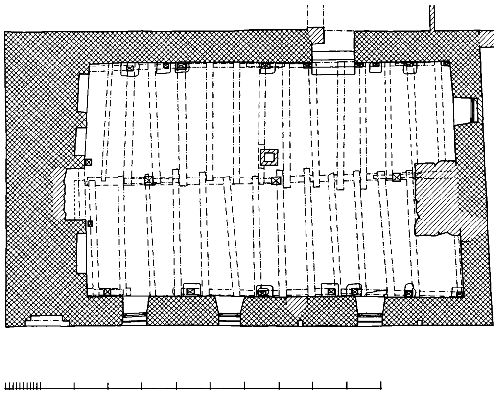
Fig. 6. Plan af kælder i mål 1:100. Opmålt nov. 1979 af Jørgen W. Overby. Skraering på grundlag af opmåling af forf. nov. 1978. Sammentegnet af Søren Gottfred Petersen.
