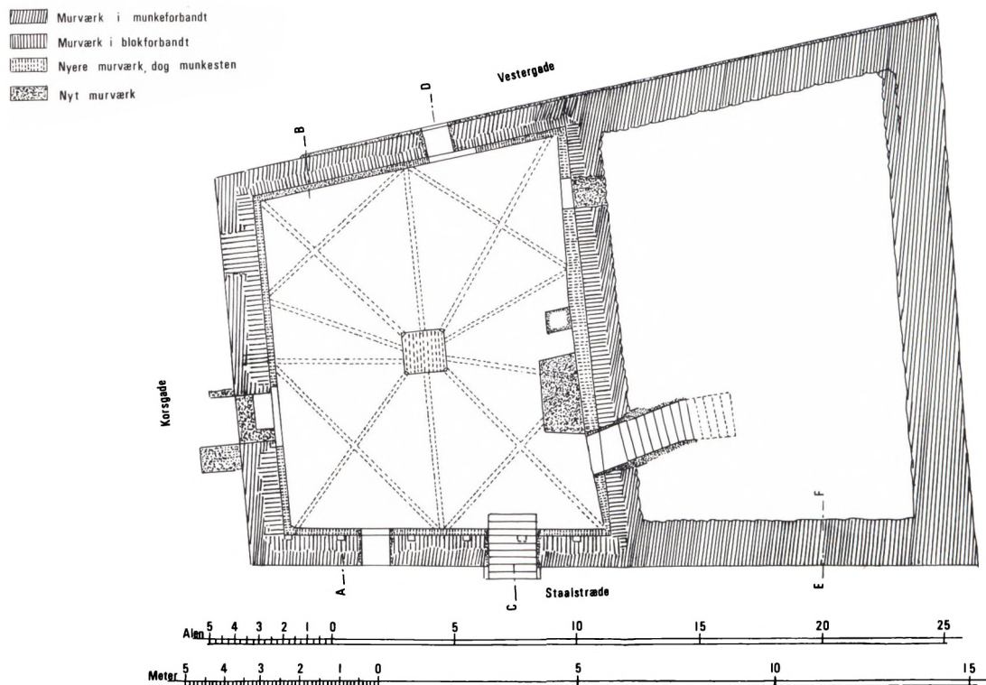
Fig. 4. Kælderplan. Opmåling af Aage H. Mathiesen 1897.
