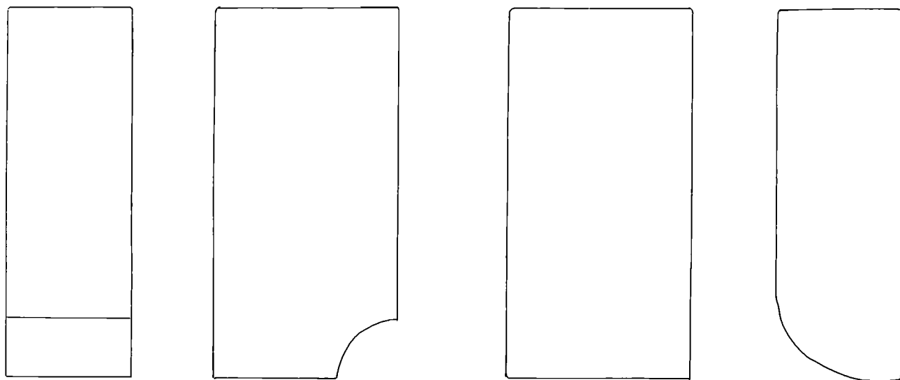
Fig. 9. Formsten. Til højre: med hulkel, fundet i 1. stokværk. Plan og side. Til venstre: med kvartrund profil, fundet i 2. stokværk. Side og plan. Mål 1:4. Opmåling af Aage H. Mathiesen.
