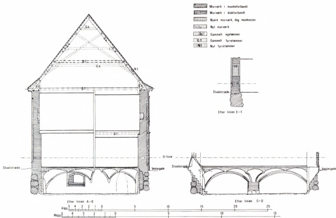
Fig. 7. Tværsnit og tagværk. Opmåling af Aage H. Mathiesen 1897.
