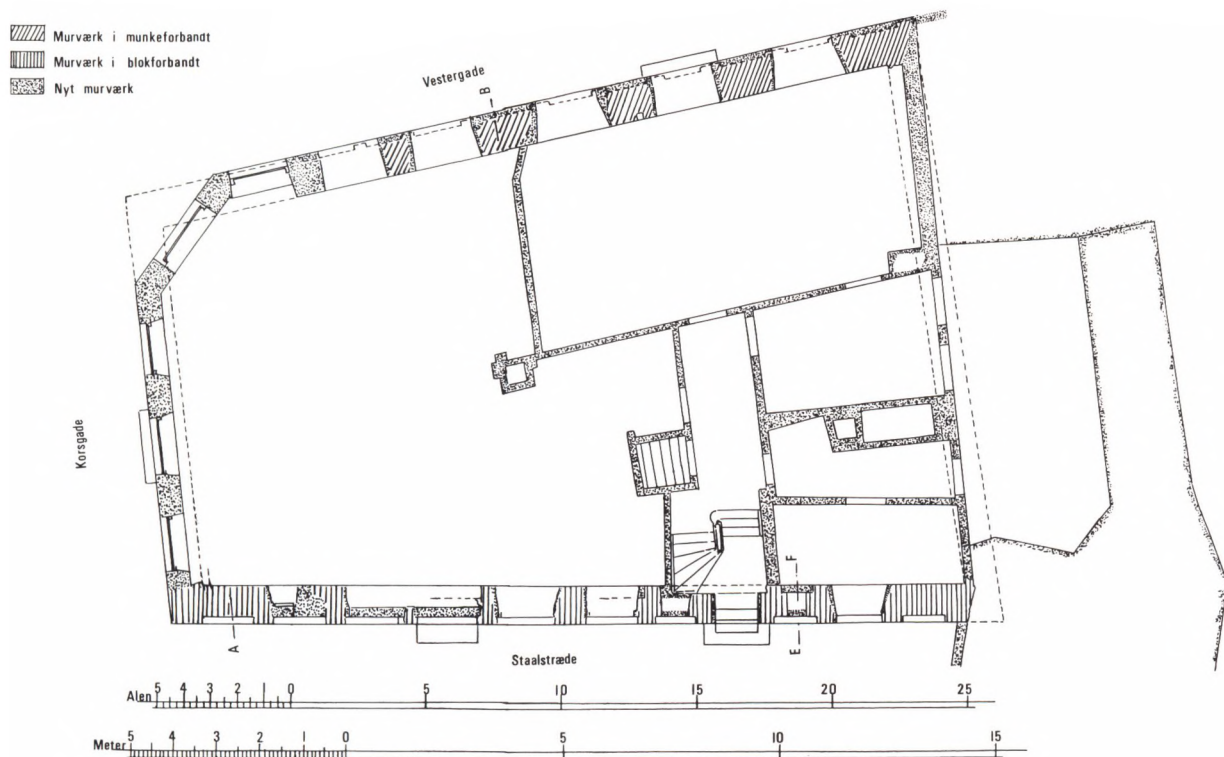
Fig. 5. Plan af 1. stokværk. Opmåling af Aage H. Mathiesen 1897.
