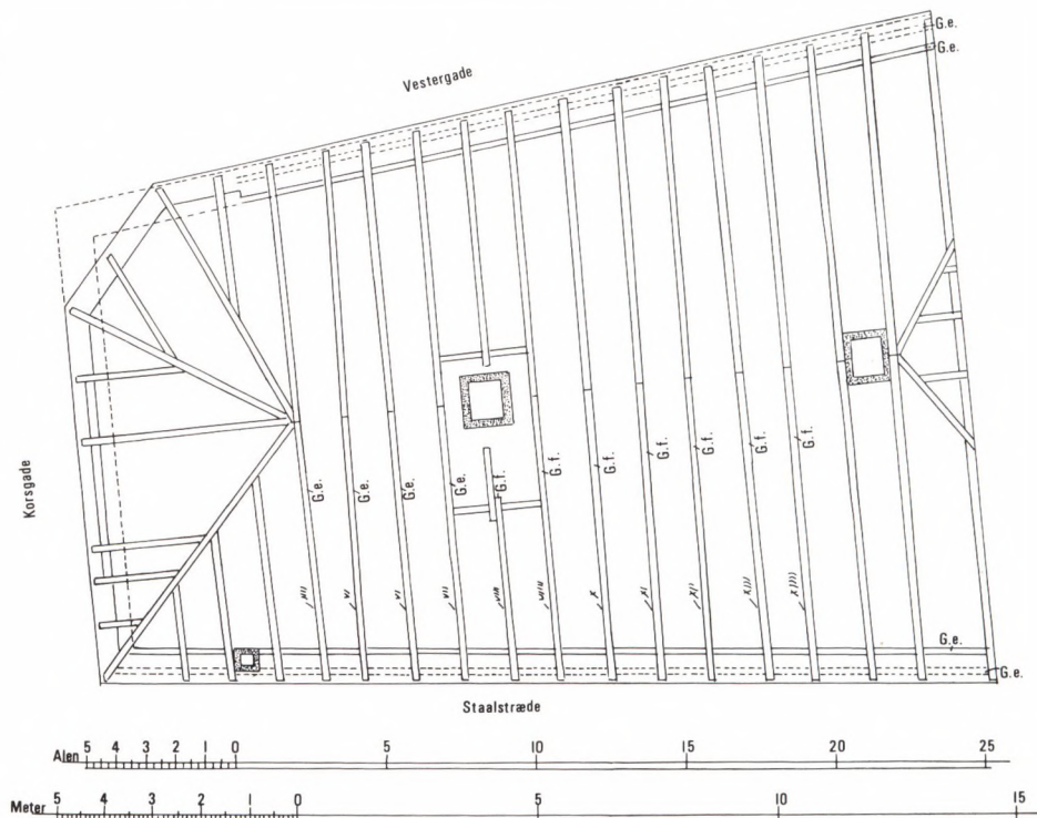
Fig. 8. Tagværk. Opmåling af Aage H. Mathiesen 1897.
