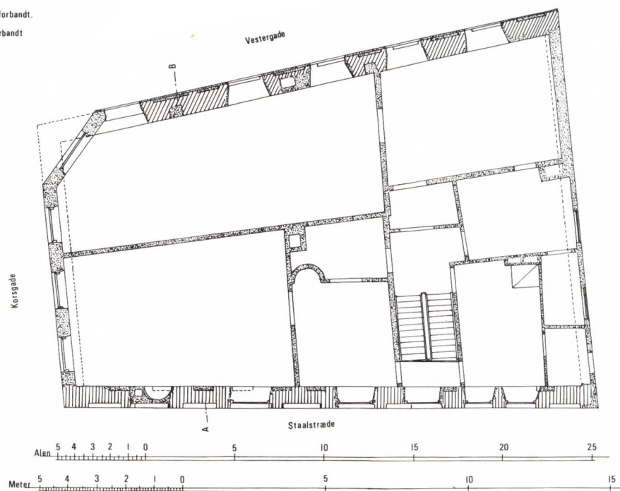
Fig. 6. Plan af 2. stokværk. Opmåling af Aage H. Mathiesen 1897.
