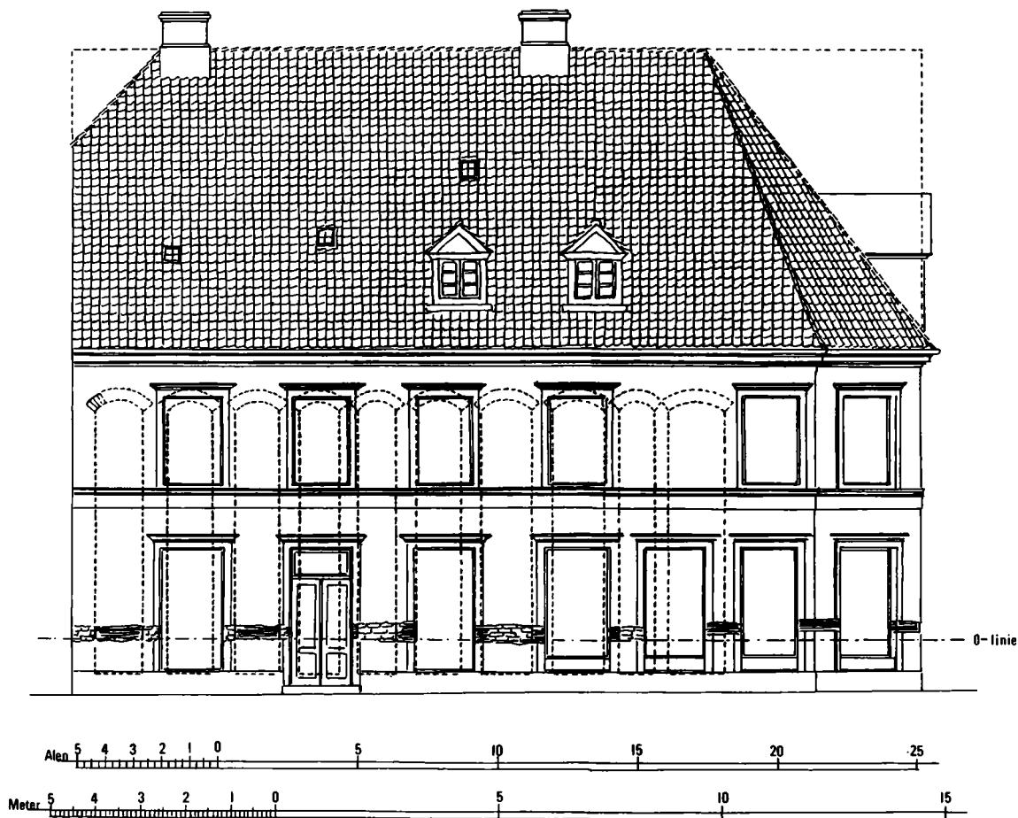
Fig. 2. Facaden mod Vestergade. Opmåling af Aage H. Mathiesen 1897.
