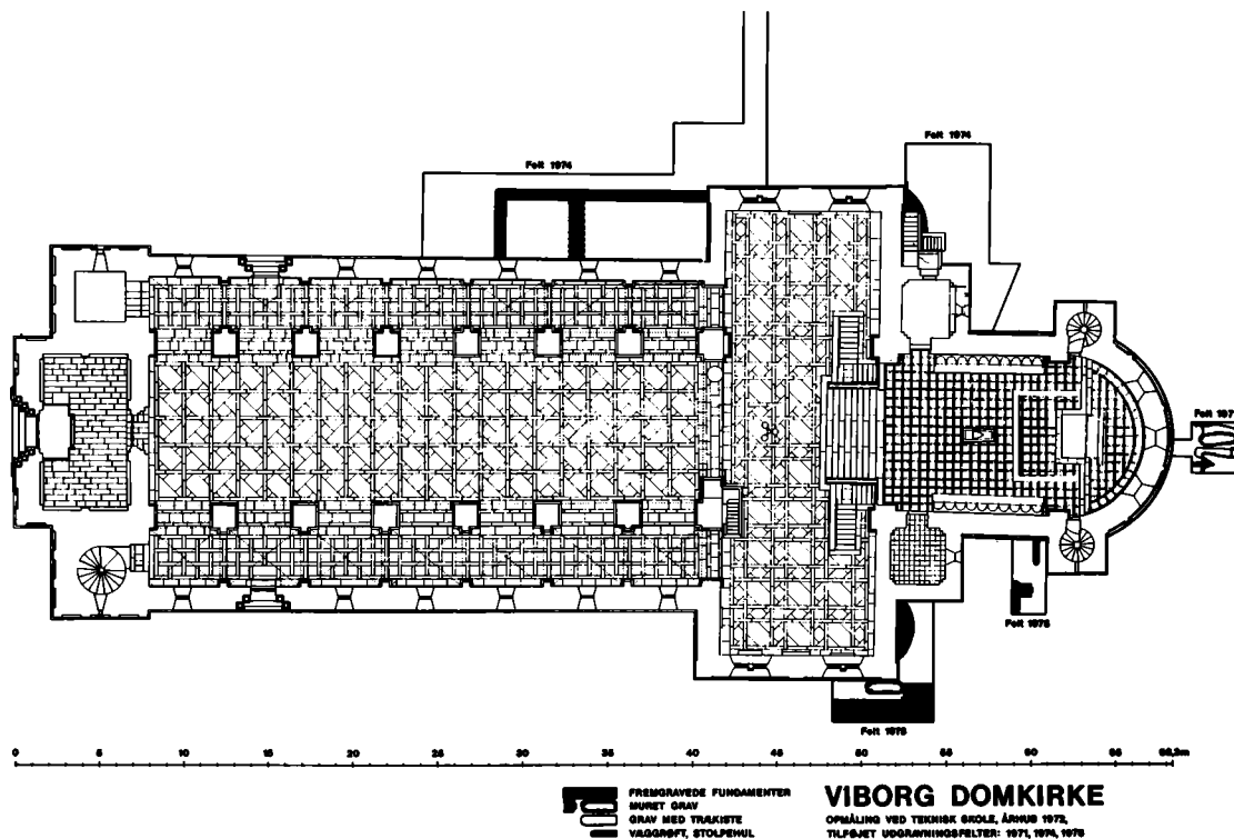
Fig. 23. Plan af Domkirken efter restaureringens færdiggørelse. Opmåling ved Århus Tekniske Skole 1971. 1859-forslagets 6 søjler i portalen er genindført. Mønsteret i kirkens indre er gulvet i kalksten lagt efter reparationsarbejdet i 1950-erne. Mål 1:500. Originalen i Domkirkens arkiv.
