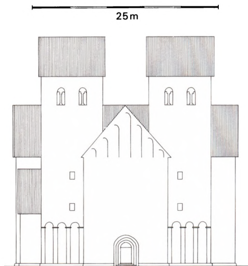
Fig. 30. Rekonstruktion af Domkirkens vestfront som den kan have set ud efter sin første færdiggørelse i begyndelsen af 1200-årene. Meget er usikkert som højden af midtpartiet og den deri siddende portals nøjere udformning. Ligeledes er tårnenes tagudformning helt hypotetisk. Men hovedindtrykket må nærme sig det rigtige. Efter tegning i Vellev 1981. Mål 1:500.
