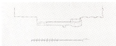
Fig. 10. Plan af fremgravede fundamenter ved Domkirkens vestfront. Mål 1:500. Opmåling ved Tholle 1865.
