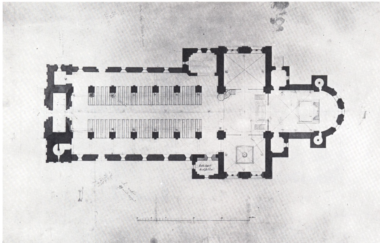
Fig. 21. Nebelongs restaureringsforslag 1859 – B2 – af Domkirken. Bemærk tilføjelserne i blyant, specielt forlængelsen af vestfremspringet. De to kapeller i nord og syd udgik ved den endelige genopførelse. Mål 1:500. Originalen på Landsarkivet i Viborg.
