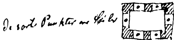
Fig. 14. Plan af Domkirkens sydvesttårn i højde med de fundne vinduer. Principskitse af Tholles i brev til svigerfaderen 1869.
