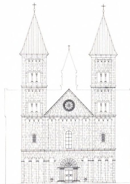
Fig. 9. Domkirkens vestfront i dag. Mål 1:500. Opmåling 1971 ved Århus Tekniske Skole. Originalen i Domkirkens arkiv.
