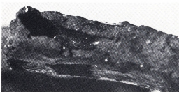
Fig. 21. Korpusskåret kat. 15, den øverste brudkant set ovenfra. I denne ses hullet efter stenen, som er sprængt ud under brændingen, samt glasuren, der er flydt ind i bruddet. Hullet måler 1 cm i længden. Foto: Preben Dehlholm.
