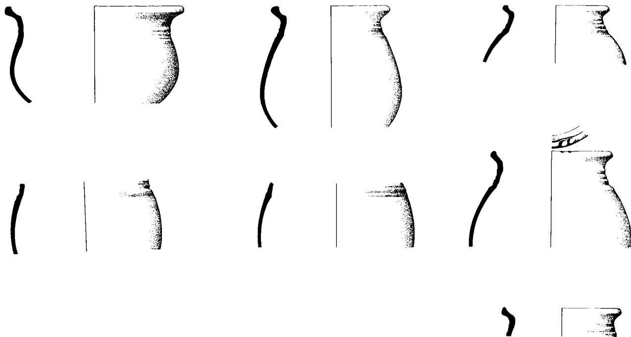
Fig. 4. Skår af gråbrændte kuglepotter, fundet i Ribe domkirke sammen med kanderne kat. 9-12. 1:4 NM2 D 7902. Opmåling og tegning: Orla Svendsen.
