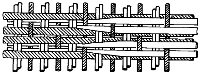
Fig. 7. Skematisk fremstilling af en 2-skuds samitumvævning. Tegningen viser en opsætning med 2 hovedkædetråde og 1 bindekædetråd. Endvidere ses hvordan de 2 skudtråde i forskellig farve bytter plads i et indslag, således at et mønster fremkommer. Efter Riboud 1976.
