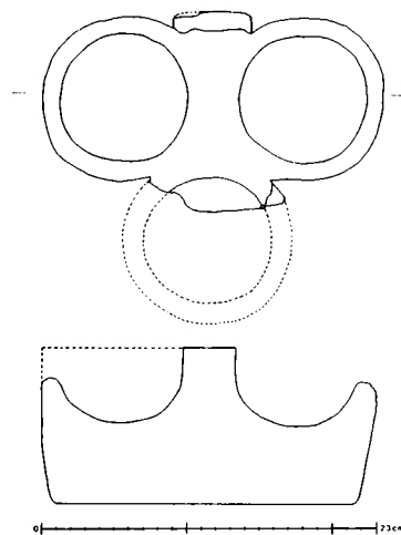
Fig. 7. Lampe fra Ribe. Opmåling: Ellen Gottliebsen 1979.
