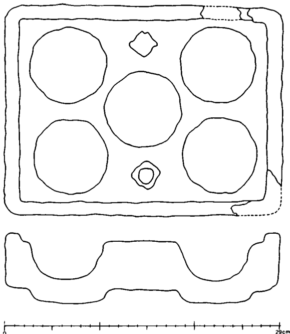
Fig. 13. »Æbleskivepande« fra Hem. Opmåling: Birgit Als Hansen 1980, tegning: Ellen Gottliebsen 1980.
