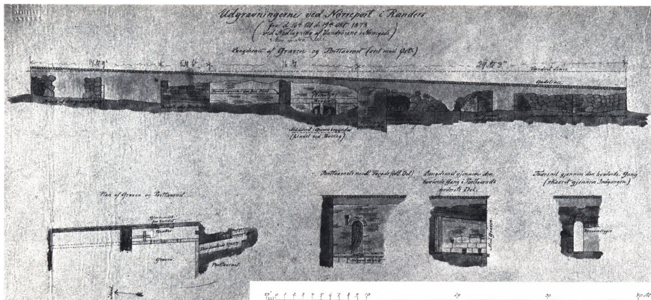
Fig. 5. Randers Nørreport. Opmåling af arkitekt Uldall 1873 på Nationalmuseets anden afdeling. Opmålingerne foreligger trykt i en let forenklet udgave i Uldalls egen rapport fra undersøgelseerne i Samlinger til Jydsk Historie og Topografi, 1912.
