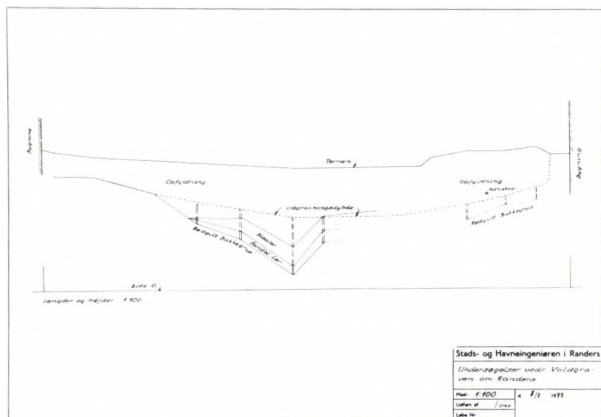
Fig. 10. Snit gennem Randers bys grav på matr. nr. 775. Den øverste del er fremkommet ved gravning, den nederste del ved borer. Afstanden mellem bygningerne er ca. 25 meter. Snittet er set mod nord. Opmåling på Nationalmuseet II.
