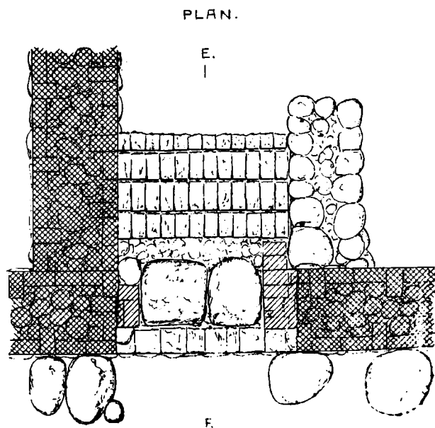
Fig. 2. Eksempel på en opmåling fra Thorvald Rasmussens hånd. Plan fra rådhusets nordre trappe, der viser det øverste fliselag i trappen. Fliserne blev fjernet af Thorvald Rasmussen. Planen i Den gl. By.
