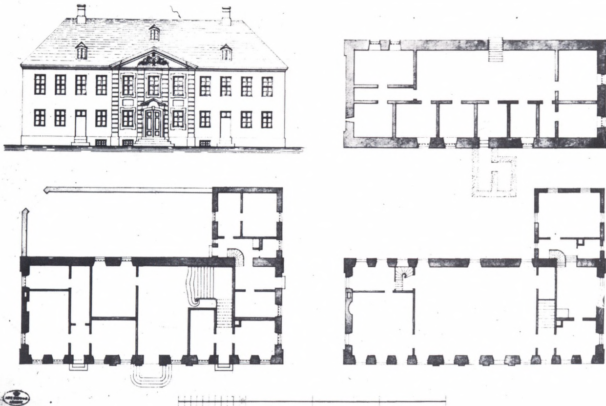
Fig. 11. Opmåling af rådhuset fra 1854, der viser huset i sin skikkelse fra ombygningen i 1750. Kunstakademiet.
