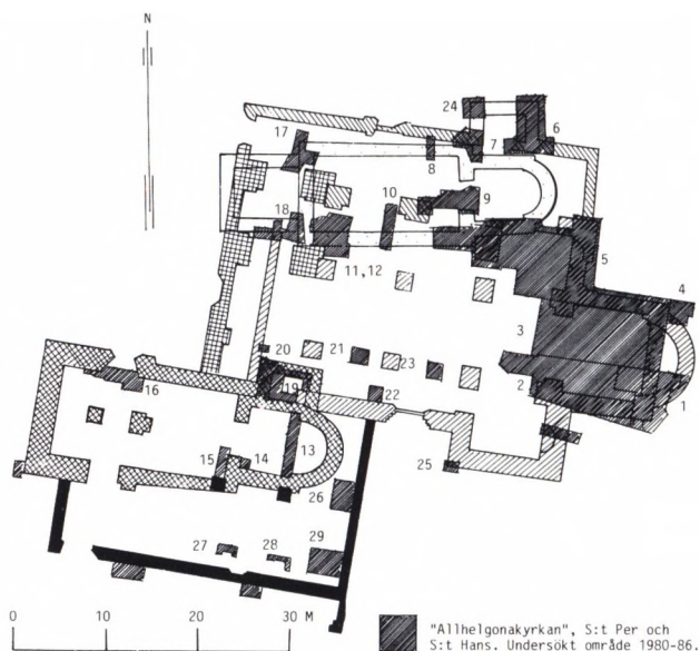
Fig. 5. »Allhelgonakyrkan«, S:t Per och S:t Hans, undersökt område 1980-86. Ritning E Swanström 1986.
