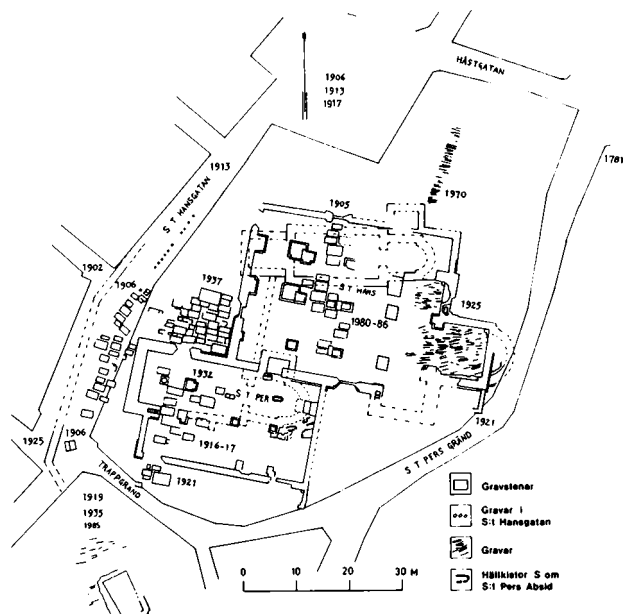
Fig. 3. Plan över undersökt område i och i anslutning till S:t Pers och S:t Hans ruiner i Visby. Ritning efter H Wideen 1943, kompletterad av E Swanström 1986.
