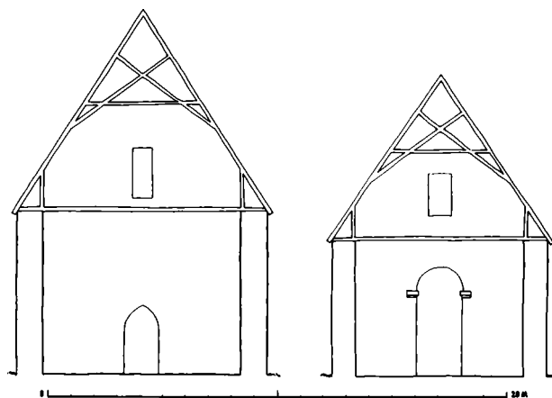
Fig. 4. Finnøy kirke til venstre, Sørbo kirke til høyre. Tverrsnitt i skipet sett mot vest. Takstolen rekonstruert.
