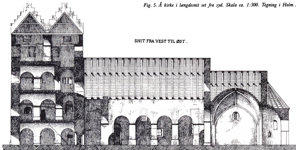
Fig. 5. Å kirke i længdesnit set fra syd. Skala ca. 1:300. Tegning i Holm 1878.
