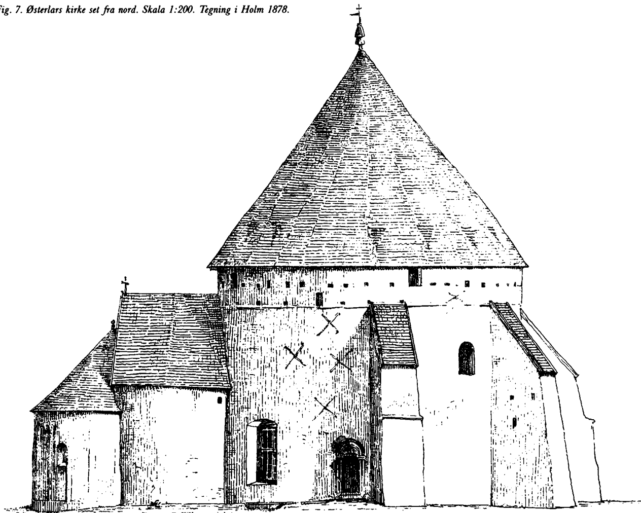
Fig. 7. Østerlars kirke set fra nord. Skala 1:200. Tegning i Holm 1878.
