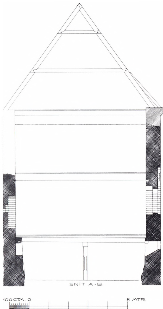
Fig. 21. Snit gennem gavlløngen set mod syd. Mål 1:100.
