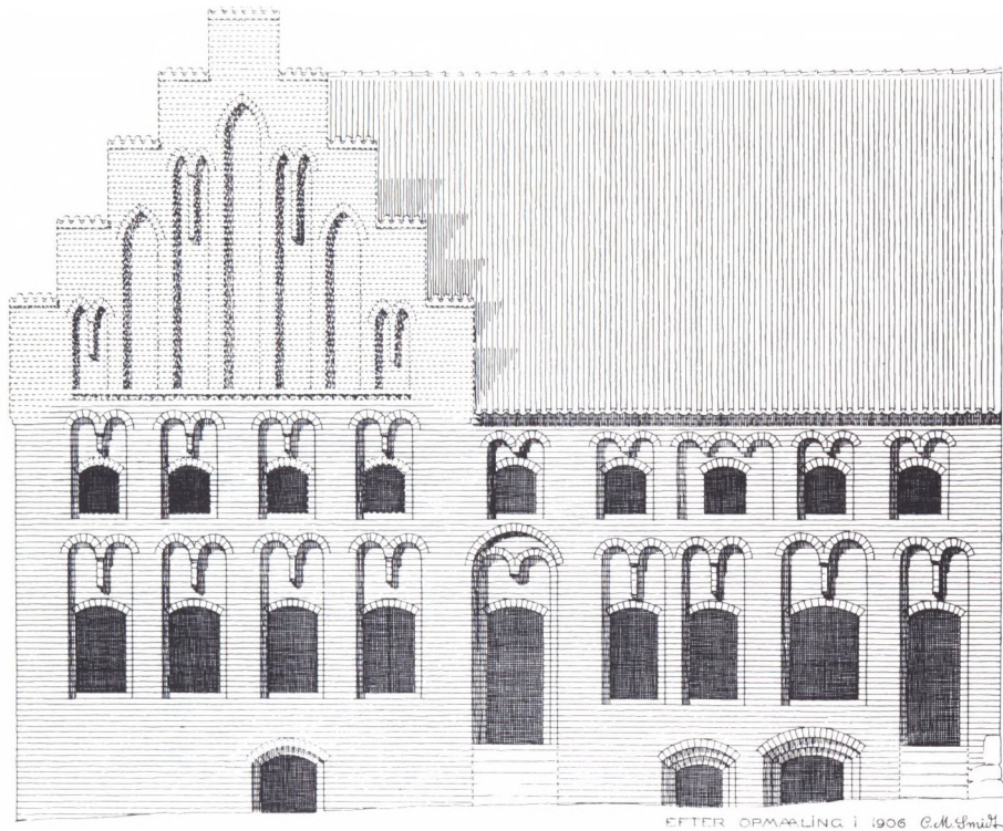
Fig. 20. Rekonstruktion af facaden mod Mathiasgade. Mål 1:150.
