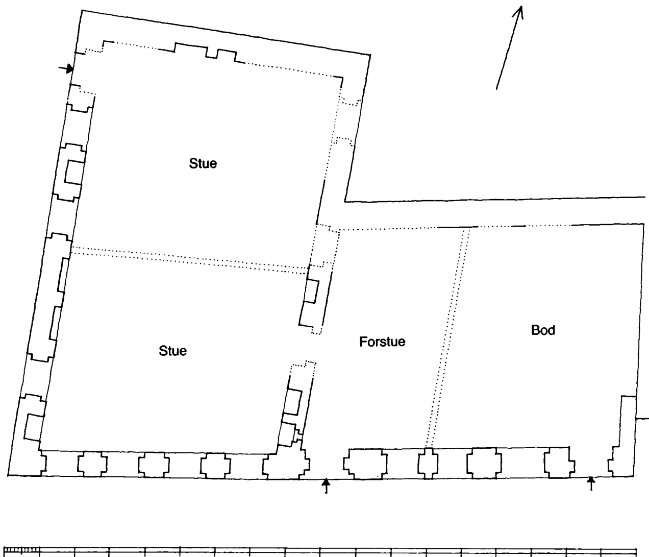
Fig. 38. Stueetagens ruminddeling, som den kan have set ud ved husets færdiggørelse. Bodan med egen indgang mod øst i sidelængen har nok været beregnet til udlejning. Forstuen kan muligvis have haft en tværdeling, så den bageste del udgjorde et lille rum for sig, for eksempel beregnet til køkken. Stuen kan dog også have indeholdt trapper til overetagen. Den nordligste del af gavlhuset med egen indgang fra Mikkelsgade kan også have haft funktion af bod. I så fald må den egentlige beboelse have været indrettet i overetagen. Rekonstruktionsforsøg ved H. H. Engqvist 1982.
