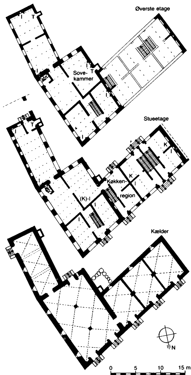
Fig. 47. Jørgen Kocks gård i Malmö. Rekonstruktionsforsøg af Sven Rosborn. Her omtegnet efter »Elbogen-Malmö fornminnesforenings tidsskrift« 1979. K = Kamin, I = Ildsted, T = Toilet.
