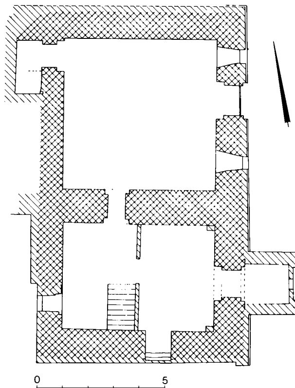
Fig. 15. Karnapgården. Plan af kælder. Opmålt af forf. 1979.
