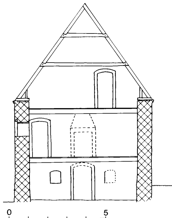
Fig. 18. Sct. Mogens Gade nr. 38. Snit i gavlhuset og indvendig opstalt af østgavlen.
