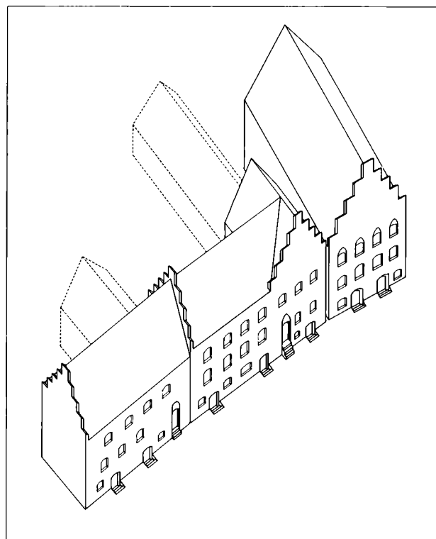
Fig. 14. Aksonometrisk rekonstruktion af nr. 5, 7 og 9. Fordelingen af døre og vinduer i de øvre etager er helt vilkårlig. Streg: Elsebet Morville.
