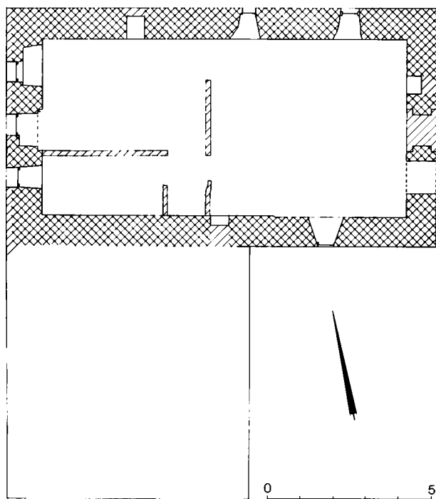
Fig. 17. Sct. Mogens Gade nr. 38. Plan af kælder. Opmålt af forf. 1979.
