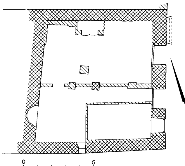
Fig. 13. Sct. Mogens Gade nr. 9. Plan af kælder. Opmålt af forf. 1978.
