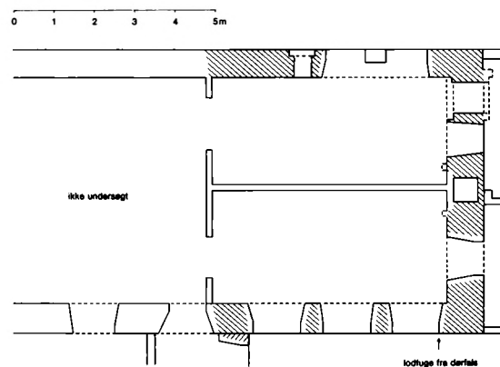
Fig. 20. Sct. Mogens Gade 38. Stueplan i gavlhusets med rekonstruktion af oprindelige forhold i østenden. Opmålt af forf. 1982. Streg: Elsebet Morville.
