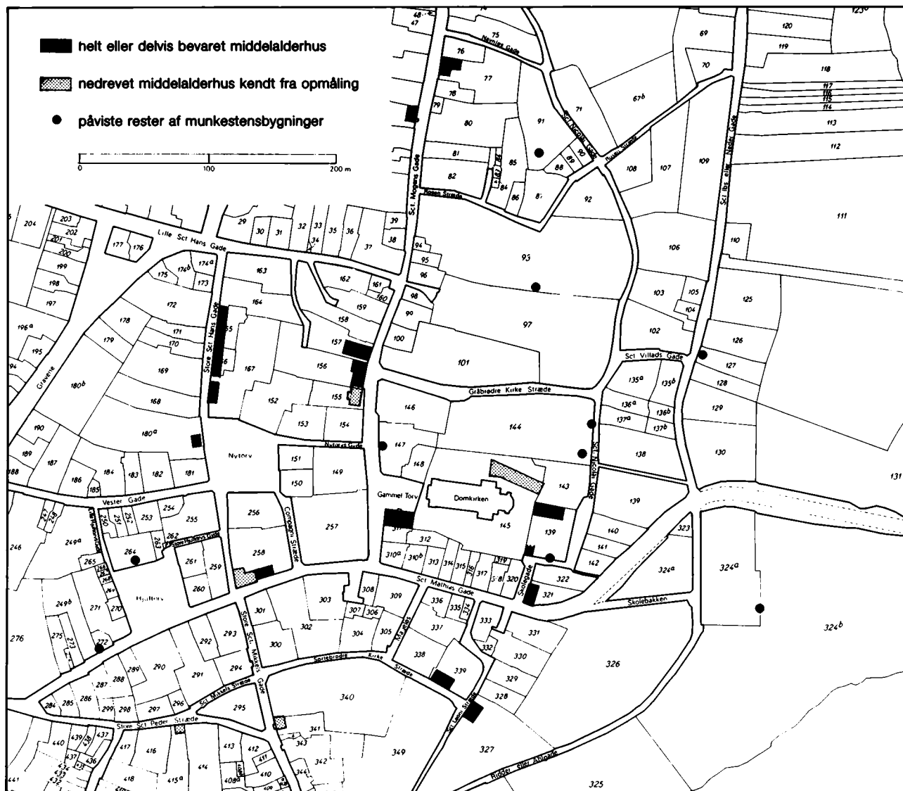
Fig. 1. Middelalderlige stenhuse i Viborg. Kortet medtager både eksisterende og kendte, nedrevne huse. Hertil kommer arkæologiske oplysninger om fund af munkestensmurværk, der dog ikke nødvendigvis i alle tilfælde behøver at stamme fra verdslige middelalderbygninger. Indtegnet på projekt Middelalderbyens grundkort med matrikelstal som i 1866.
