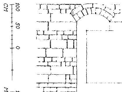
Fig. 6. Stengade 66. Afrenset parti af sidebygningens murværk mod Færgestræde med bælter af munkesten og kridtsten samt et smalt tilmuret vindue med prydskitte over det fladbuede halvstensstik. Skitseopmåling udført i 1975 af Ruth Fhær Larsen. Her gengivet i mål 1:50.
