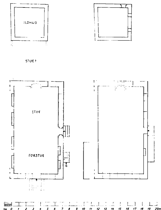
Fig. 28. Stengade 74. Oprindelig stueplan (t.v.) og salsplan (før ombygningen i 1542-43). Rekonstruktionsforsøg (HHE) tegnet på grundlag af Volmar Drosteds reviderede opmålinger og fotografier taget under restaureringen 1932-36. Mål 1:300.
