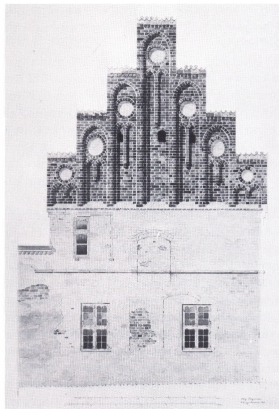
Fig. 3. Stengade 66 (Oxernes Gaard). Gavlen mod Færgestræde. Opmåling udført i 1903 af Holger Hagemann. Her gengivet i mål 1:150 efter Ældre Nordisk Architectur , 4. samling, 3. række.
