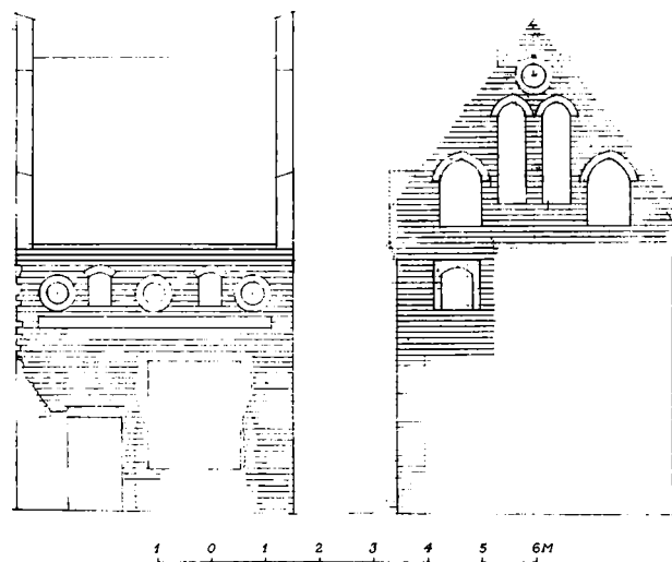
Fig. 32. Stengade 74. Ildhusets vestside og sydgavl. Tegnet (med oprindelig gesims og tag) af HHE på grundlag af Volmar Drosteds opmåling fra 1935 og fotografier taget under restaureringen (i Helsingør Bymuseum). Mål 1:150.
