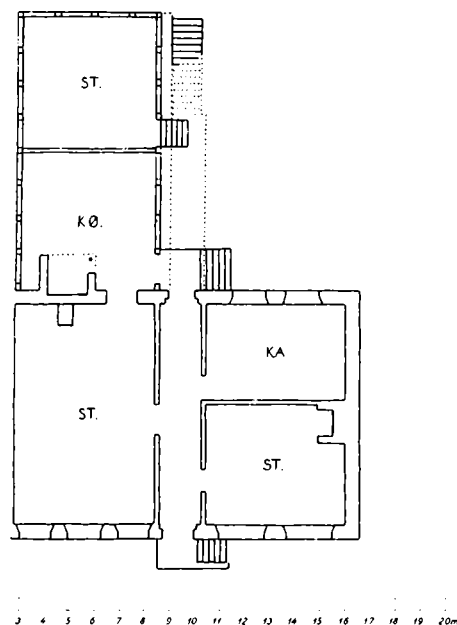
Fig. 19. Strandgade 30 på Christianshavn. Rekonstruktion af stueplan (HHE 1945) gengivet i mål 1:300. Det vinkelbyggede hovedhus med gennemgående forstuegang i gadesløjens midte og køkken i sidebygningen umiddelbart op til den store stue, som beslaglægger den ene ende af gadesløj, genfindes i en del københavnske bygårde fra tiden omkring 1600. Også i købstæderne er denne udformning af gårdenes hovedbygning såre almindelig, dog er forstuen her som oftest placeret i gadelængens ene ende umiddelbart op til indkørselsporten.
