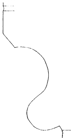
Fig. 22. Stengade 72. Forhusets kridstensgesims. Profil i mål 1:5.
