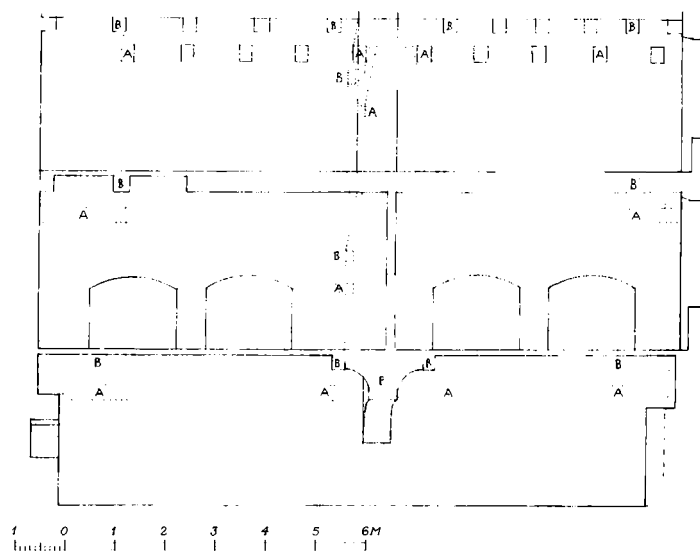
Fig. 42. Stengade 76. Den vestre langmur set indefra. Opmåling i mål 1:150 tegnet på grundlag af opmålinger og fotografier fra 1911 i Nationalmuseets 2. afdl. I overetagen ses de oprindelige (middelalderlige) bjælkehuller (mrk. A) og de nuværende bjælker fra 1579 (mrk. B). Den formodede oprindelige bjælkelagsplacering i kælder- og stueetage er vist med prikning og mærket med A. Tørmuren og de to kvartbuehælv, der bærer de ovenover liggende ildsteder, er fra 1579. Ildstederne og højdeplaceringen af skorstenshamrene før og efter David Hansens ombygning i 1579 er antydet med prikning og bogstaverne A og B.
