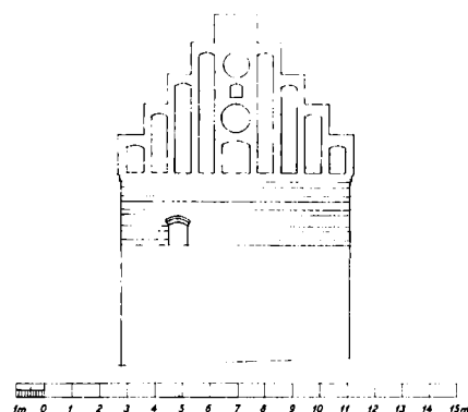
Fig. 9. Strandgade 79, som formentlig er opført mellem 1574 og 1578. Gavl mod Færgestræde. Skitse (HHE) i mål ca. 1:300.
