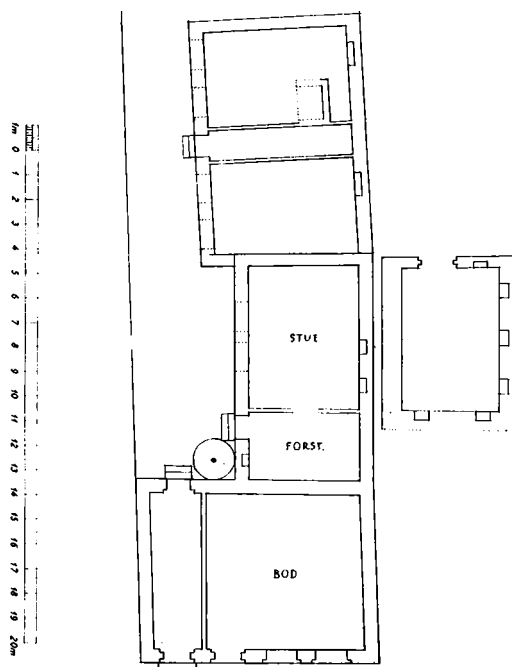
Fig. 12. Stengade 70. Stueplan med plan af sidebygningens kælder (i.h.). Rekonstruktion på grundlag af skitseopmåling og undersøgelse foretaget i 1975 og 1980 af HHE m.fl. Mål 1:300.
