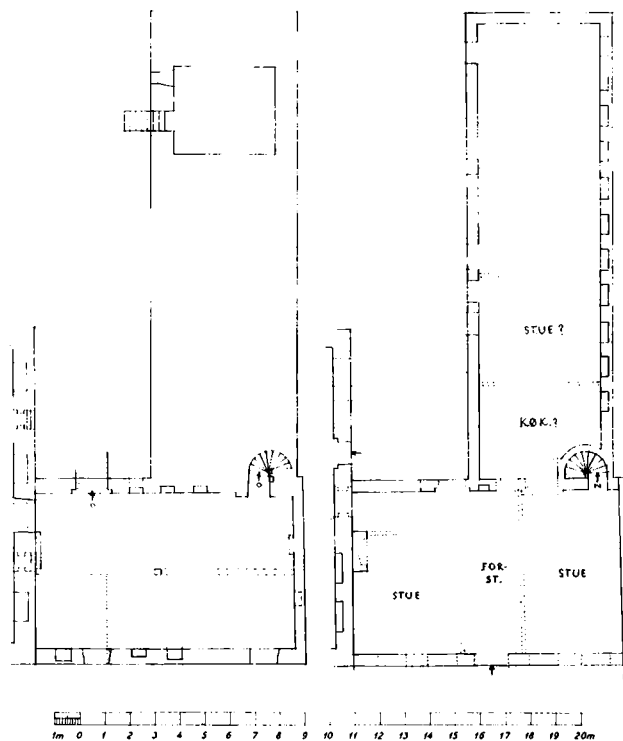
Fig. 18. Stengade 72. Opmåling af kælderplan (t.v.). Det tidligere forhus er indtegnet med prikket kontur. Til højre stueplan, rekonstruktionsforsøg. De formodede muråbninger og skillerum m.m. er angivet med prikning. Tegnet af HHE – for kældrens vedkommende på grundlag af en opmåling udført i 1975 af studerende ved Kunstakademiets Arkitektskole og for stueetagens vedkommende på grundlag af Volmar Drosteds reviderede opmåling fra 1935. Planerne er her gengivet i mål 1:300.
