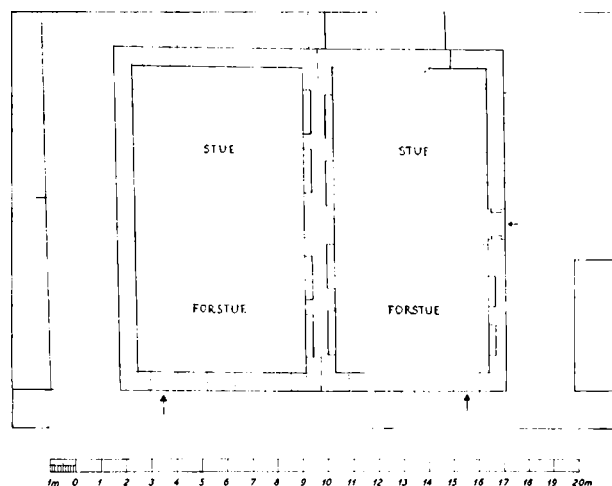
Fig. 40. Stengade 74 og 76. De to sammenbyggede gavlhuses oprindelige stueplan. Rekonstruktionsforsøg (HHE) i mål 1:300. Nicheerne i de sammenbyggede langmure har samme bredde, men en noget afvigende placering.
