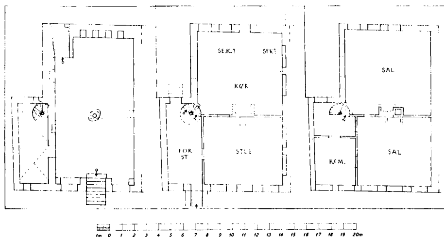
Fig. 41. Stengade 76. Opmåling af kælderplan (t.v.) og rekonstruktion af stue- og salsplan ved tiden omkring 1740 tegnet af HHE på grundlag af opmålinger (bl.a. i Nationalmuseets 2. afd.), egne iagttagelser og auktionsskøder fra 1740 og 1748. Mål 1:300. Den indretning, gavlhuset havde efter David Hansens ombygning i 1579, kan næppe have adskilt sig nævneværdigt fra den som fandtes i 1740-erne og som i øvrigt stort set endnu fandtes i 1911.
