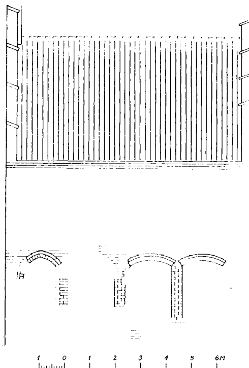
Fig. 11. Stengade 70, som formentlig er opført i første fjerdedel af 1500-årene. Den partielt afrensede gadeside. Opmåling (HHE 1980) i mål 1:150.
