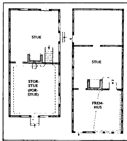
Fig. 31. Eksempler på gavlhusplaner af norrøjsk type. Til venstre Poul Pops Trefoldighedshus i Aalborg fra 1571. Til højre Korsgade 11 i Assens fra årene omkring 1570. Rekonstruktioner (HHE) i mål 1:300.
