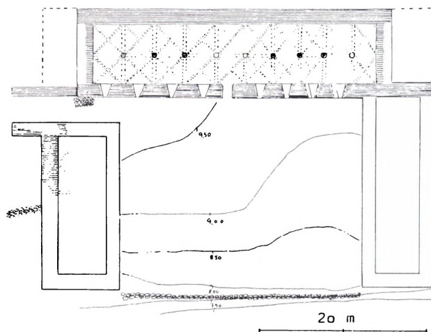
Fig. 6. Grundplan af den middelalderlige bispegård tegnet på grundlag af ældre opmålinger samt udgravningen af vestfløjen i 1976. Tegning Jørgen Nielsen, Møntergården. Kilde: Fra boplads til bispeby. Odense til 1559 s. 407.
