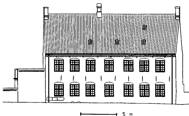
Fig. 20a. Sankt Hans præstegårds sydside mod kirkepladsen. Opmåling af Jørgen Stjernose 1941. I forhold til originalen er indsat en målestok. Kilde som fig. 17. s. 45.
