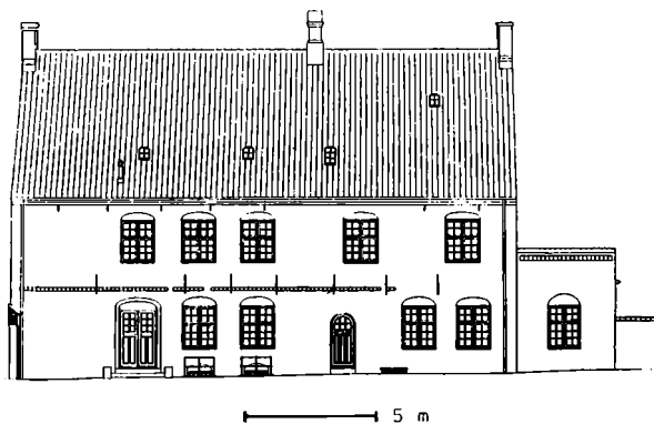
Fig. 20b. Sankt Hans præstegårds nordside. Opmåling af Jørgen Hvenegaard Lassen 1941. I forhold til originalen er indsat en målestok. Kilde som fig. 17. s. 45.
