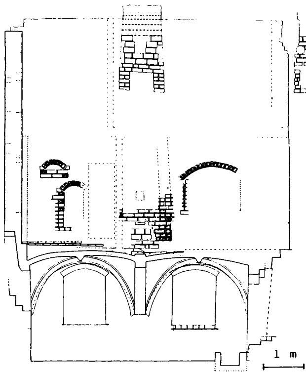
Fig 23. Vestgavlens inderside, Overgade 3. I kælderen ses den murede kumme og i de andre stokværk ses skorstenen med to kaminer. Kilde: F. Grandt-Nielsen, To middelalderlige stenhuse i Odense. Fynske Minder 1970 s. 147. I forhold til originalen er indsat en målestok.
