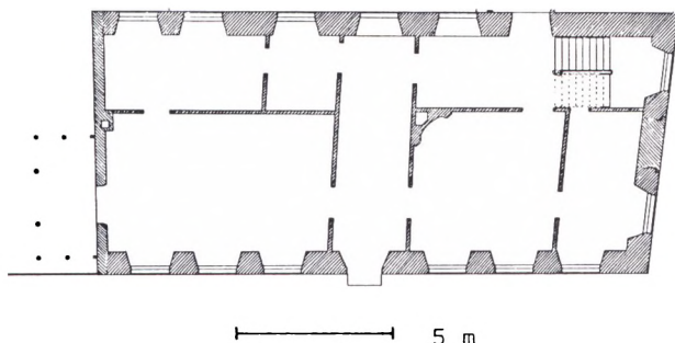
Fig. 17. Sankt Hans præstegård. Plan af 1. stokværk opmålt af N. Jacobsen i 1905. Kilde: Victor Hermansen, Sct. Hans Præstegaard i Odense, Fynske Aarbøger II , Odense 1942-1946, s. 30. I forhold til originalen er indsat en målestok og tilbygningerne fjernet.
