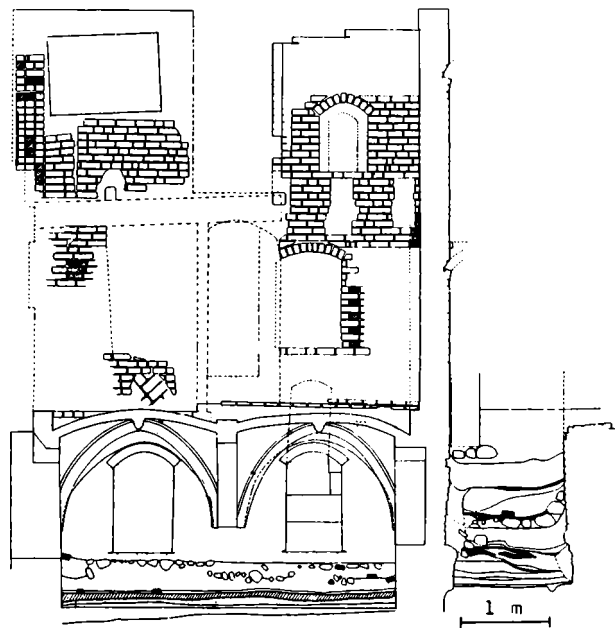
Fig. 24. Overgade 3. Sydmurens inderside. T.h. ses slippen mellem de 2 huse. De ældre lag ses både i kælderen og i slippen mellem husene. Kilde: F. Grandt-Nielsen, To middelalderlige stenhuse i Odense. Fynske Minder 1970 s. 145. I forhold til originalen er indsat en målestok.
