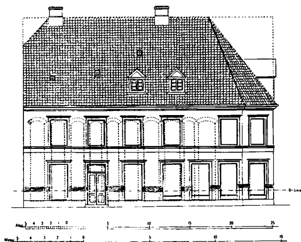
Fig. 32. »Priorgården« Vestergade 1. Facaden mod Vestergade opmålt af Aage H. Mathiesen 1897. Kilde: Ebbe Hædersdal, Priorgården i Odense , Hikuin 7, Højbjerg 1981, s. 150.
