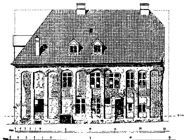
Fig. 33. »Priorgården« Vestergade 1. Facaden mod Stålstræde opmålt af Aage H. Mathiesen 1897. Kilde: Ebbe Hædersdal, Priorgården i Odense , Hikuin 7, Højbjerg 1981, s. 151.
