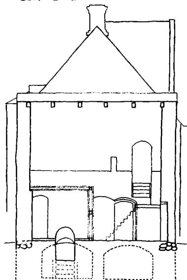
SNIT C-C
