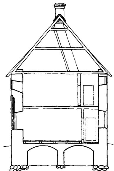
SNIT B-B
