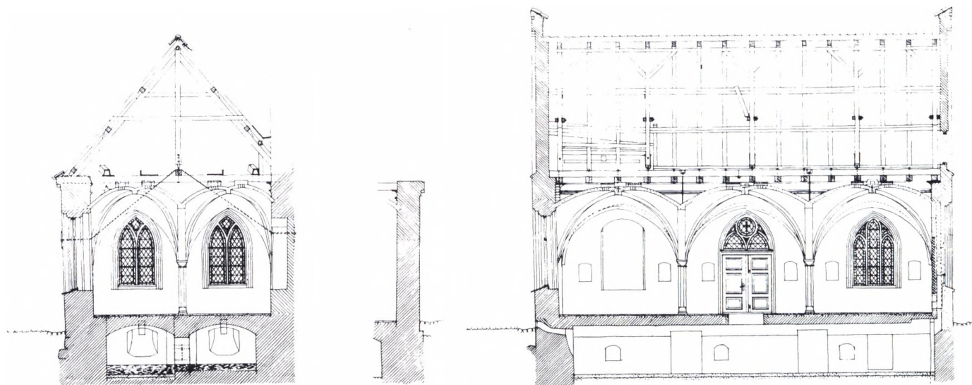
Fig. 13. Sydfløjen, tværsnit mod vest og nord 1916-1973. Hvælv og middelalderlig overetage fjernedes 1783, da en ny etageinddeling etableredes. Denne sløjfedes atter 1863 (arkitekt Chr.Hansen), da hele bygningen indrettedes til ligkapel med gipset loft, de oprindelige vinduer mod syd og vest genåbnedes og der nyoprettedes to tilsvarende vinduer i nordmuren, mens porten placeredes i østgavlen, der nymuredes med kamtakker. I 1916 (arkitekter Mogens Clemmensens og E.Vilh. Olsen) genopførtes hvælvene og porten flyttedes til nordmurens midte. Ved restaureringen 1972-73 (arkitekter Rolf Graae og Erl. Jessen) sløjfedes port og vindue i nordmuren, mens til gengæld den store niche blev gennembrudt for oprettelse af en forbindelse til vestfløjen. Målt og tegnet af I.Arthur-Nielsen 1970. Mål 1:200.
