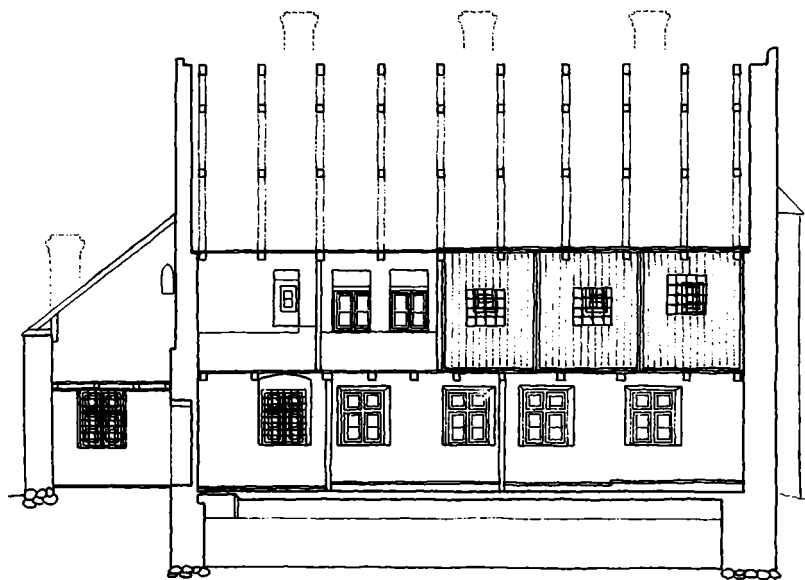
SYDFACADE SET I NDEFRA SØIT E-E
