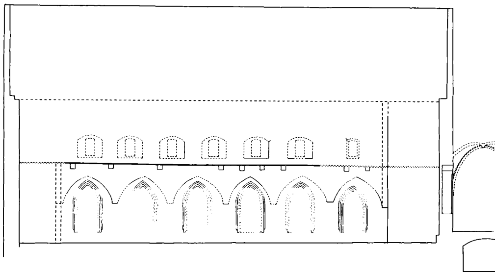
Fig. 10. Vestfløjens gårdfacade set indefra. T.h. tværnsnit af sydfløjen (refektoriet). Rekonstruktion efter opmåling af L.Arthur-Nielsen 1970, suppleret 1970 af H.G. Tegnet af Anett Andersen 1990. Mål 1:200.
