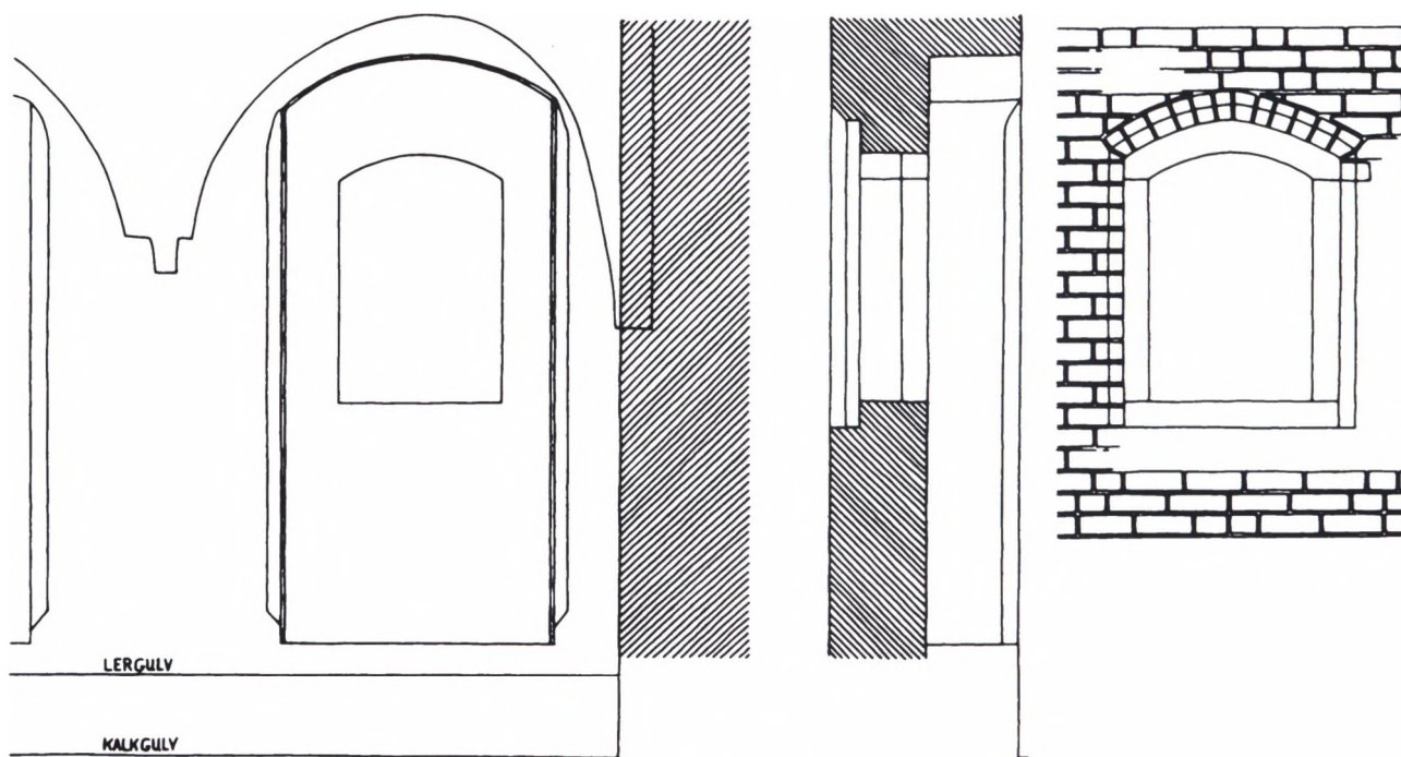
Fig. 8. Vinduesniche i vestfløjens vestvæg. Målt af L.Arthur-Nielsen 1970. Tegnet af Tina Hansen 1991. Mål 1:40.
