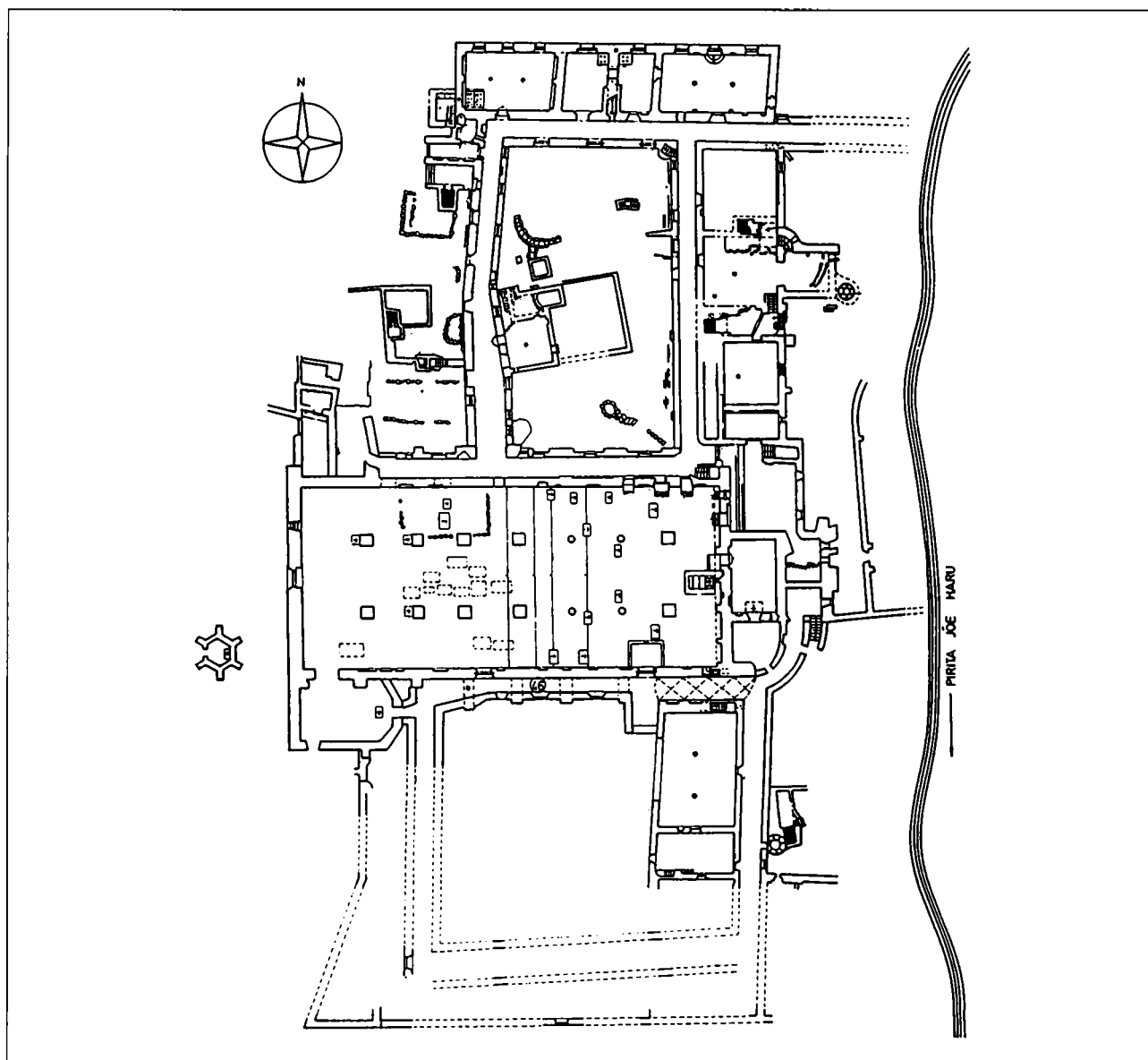
Fig. 13. Grundplanen över klostret i Pirita.
