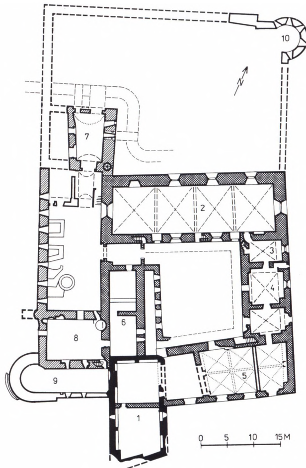
Fig. 3. Grundplanen över klostret i Padise.
