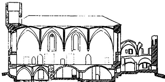
Fig. 4. Klostret i Padise. Längdsnitt av norra flygeln.
