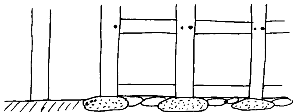
Fig. 1. Skitse af hvordan forskellige bindingsværksvægge kunne være funderet i Skast Herred i 16-1700-tallet, efter oplysninger fra tingbøgerne.
