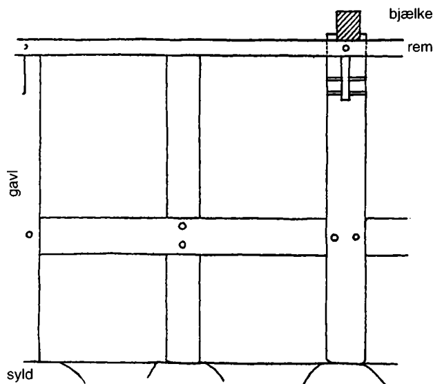
Fig. 2. I 1946 fandt Nationalmuseet ved bondegårdsundersøgelserne i Vestjylland et enkelt fag bindingsværk i Skast herred, i en gård i Størsbøl, V.Ny-kirke s. Her var bevaret to vægstolper af egetræ med vægrem samt en overlagt bjælke. Bjælken og stolperne havde indvendig spor af indtappede skråbånd, der førhen var ret almindelige også i denne egn. Vægstolperne stod på sten og der var både en løsholt og to »dockstænger«, faget var i øvrigt udmuret med brændte teglsten. Skitse af D. Yde Andersen og rentegnet af Ib Steen-Jensen. Nationalmuseet N.E.U. 10.172.
