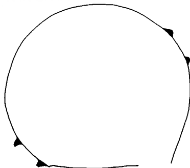
Fig. 8b. Vandret tværsnit af armringen fig. 8.
