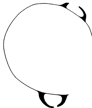
Fig. 9a. Vandret og lodret tværsnit af armringen fig. 9.
