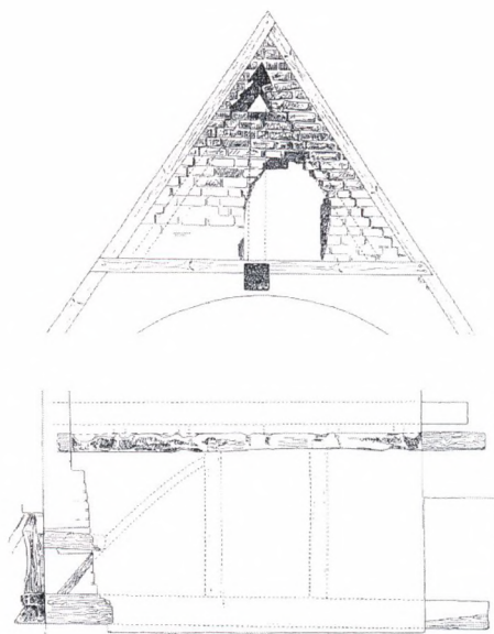
Fig. 5. Ryde Kirke, Lolland søndre Herred, Maribo Amt. Tværsnit af kor set mod vest og længdesnit set mod syd. 1:100. Tøndehvælvet der antydes fjernet i snittet er oprindeligt. Efter Danmarks Kirker, målt af Mogens Clemmensen.
