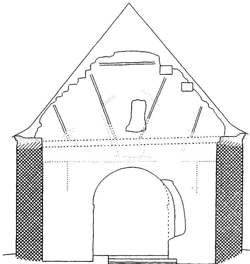
Fig. 3. Fejlslev Kirke, Horns Herred, Frederiksborg Amt. Tværsnit ved triumfmurens vestside med spor efter skibets og korets (punktet) oprindelige tagværker. 1:100. Bemærk den lave taghældning og aftrykket efter rygningbrædderne i koret. Efter Danmarks Kirker, tegning: Henrik Jacobsen.
