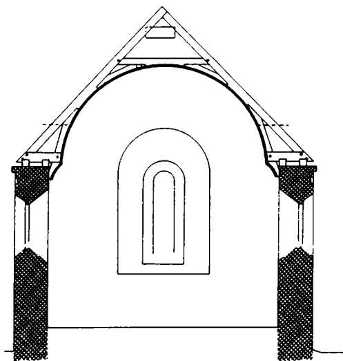
Fig. 6. Skørpinge Kirke, Vester Flakkebjerg Herred, Sorø Amt. Snit gennem kor, set mod øst, opmåling og rekonstruktion. 1:100. Efter Danmarks Kirker, målt af C. G. Schultz.
