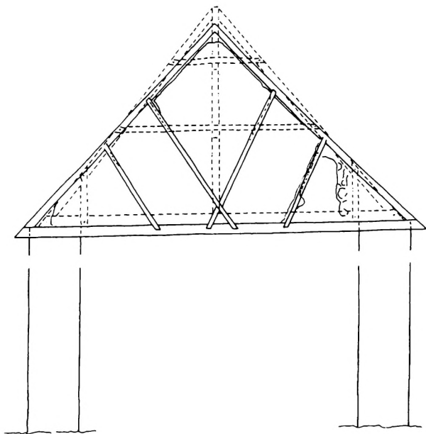
Fig. 4. Bjergsted Kirke, Skippinge Herred, Holbæk Amt. Tværsnit ved triumfmurens vestside. Oprindeligt tagværk indtegnet efter bevarede spor (nuværende tagværk stiple). 1:100. Efter Danmarks Kirker; opmåling: Thora Fisker.
