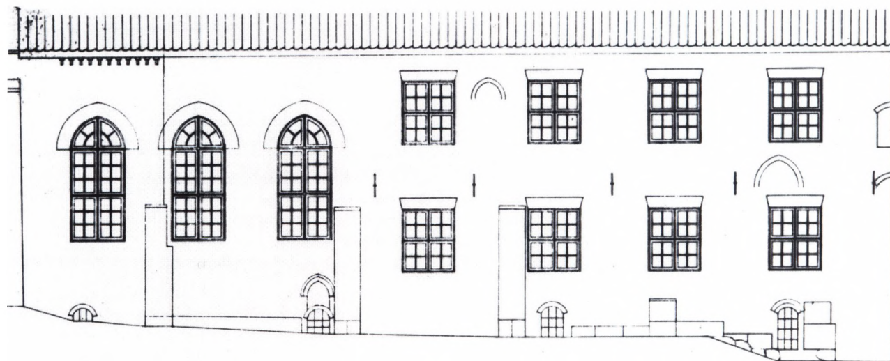
Fig. 16. Opmåling af den sydlige del af vestfløjens facade mod øst inden restaureringen i 1880'erne. Kunstakademiet, Samlingen af Arkitekturtegninger.
