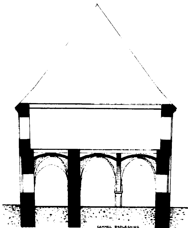
Fig. 24. Snit på tværs af Skolefløjen. Til venstre klostergangen, til højre den sydligste af de tre rum, som formentlig har tjent som sakristi. Opmålt omkring år 1900. Kunstakademiet, Samlingen af Arkitekturtegninger.
