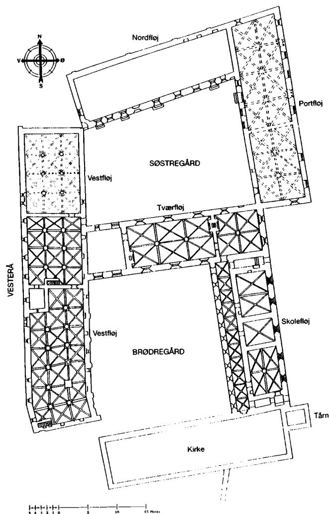
Fig. 4. Grundplan af det fuldt udbyggede Helligåndskloster ved Reformationen. Kirken, der ligger som sydføj i anlægget, er indtegnet efter de få mål, som kendes. I vestfløjen er kælderens hvælvslagning angivet, i de øvrige fløje underetagerne. Ikke bevaret hvælvslagning er markeret med stiplede linie. Tegning: Jan Slot-Carlson og Leif Plith Lauritsen.
