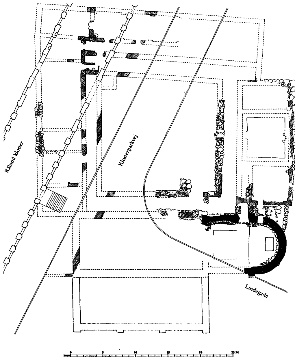
Fig. 10. Grundplan af gråbrødrekløstret i Kalundborg. Ved at kombinere forskellige forskeres ældre undersøgelser fra 1948, 1961, 1964 og 1975 er det for nylig lykkedes at få overblik over klosterplanen. Samtidig fremgår det klart, at anlegget er et resultat af et ganske kompliceret byggerforløb med mange faser i nordvesthjørnet og med en flytning af østfløjen. Tegning: Mogens Vedsø 1995 (efter Danmarks Kirker).
