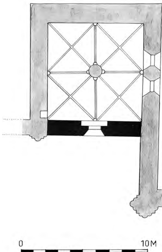
Fig. 6. Författarens tolkning av sakristia 2-skedet. Ritning: Gabriela Buschmann-Martin 2002.
