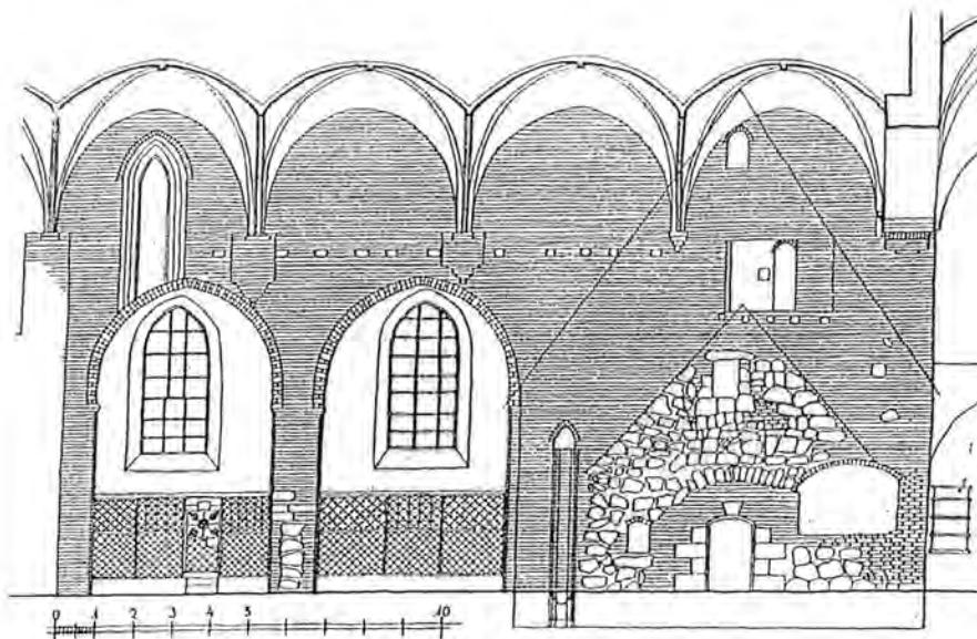
Fig. 4. Den östra delen av långhusets nordvägg. Efter Rinne 1941.
