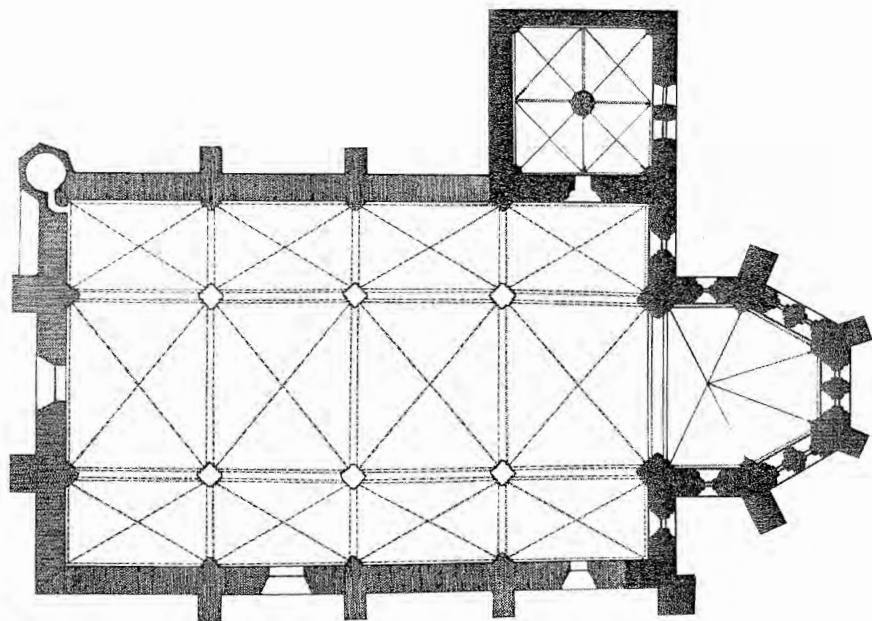
Fig. 5. Iikka Kronqvists tolkning av sakristia 2-skedet och av den äldre planen för uppförande av en tegelkyrka. Efter Kronqvist 1948.
