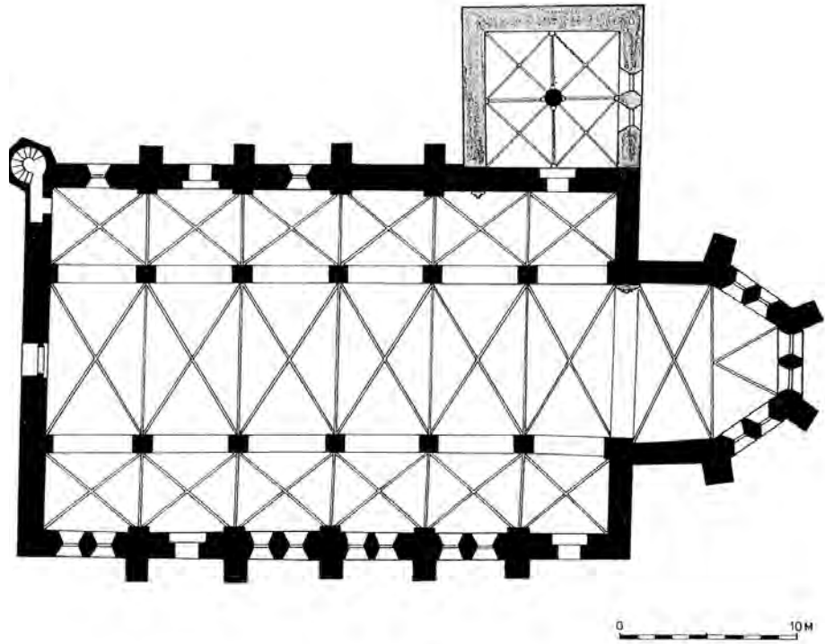
Fig. 7. Principskiss av den förverkligade tegelkyrkans plan. Detaljerna fritt efter J. Rinne och I. Kronqvist. Rättning: Gabriela Buschmann Martin 2002.
