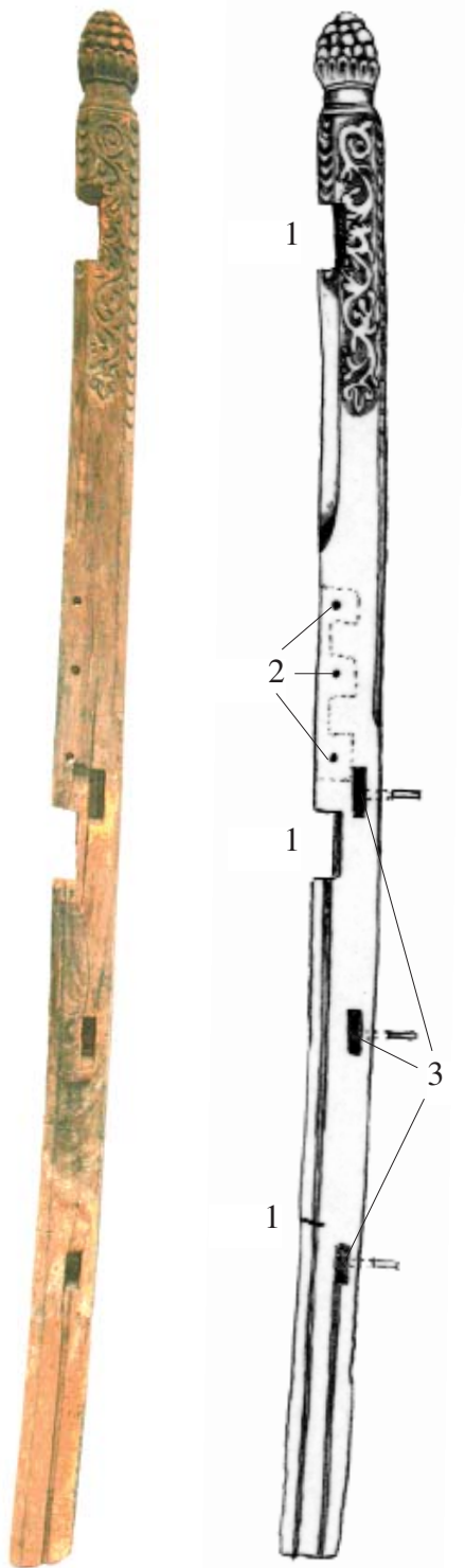
Fig. 5. Sengestolpe af egetræ med udskæringer. Længde: 220 cm, tværmål: ca 7,5 x 9 cm. Foto og tegning: Mette H. Søvsø.
